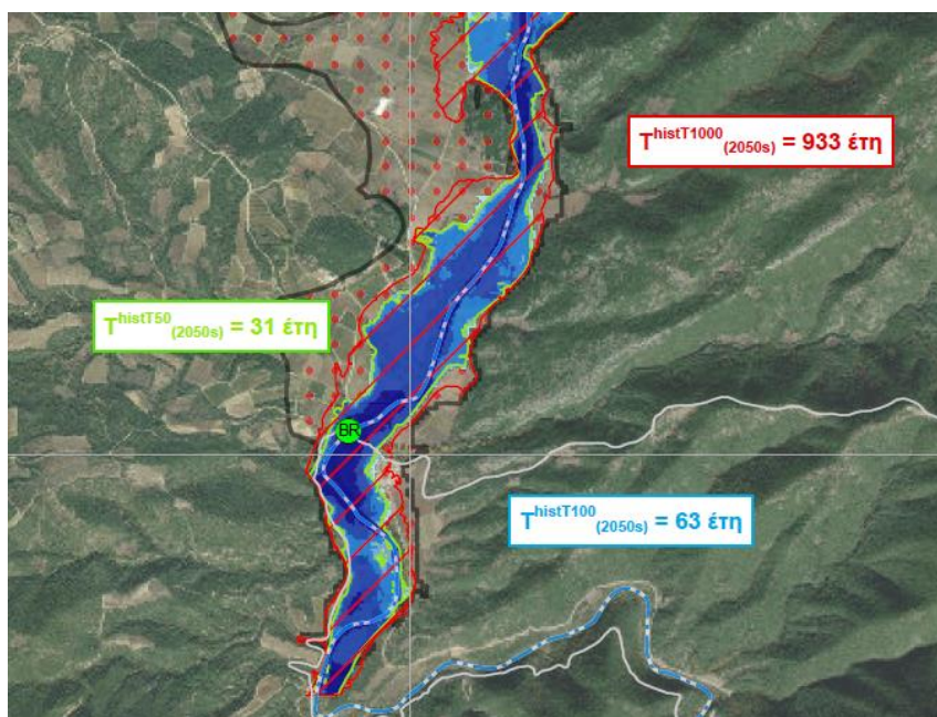
Σχήμα 4-16: Αντιστοίχιση της περιόδου επαναφοράς σε συνθήκες κλιματικής αλλαγής εντός των Χαρτών Επίδρασης Κλιματικής Αλλαγής, παράδειγμα εφαρμογής στο ΥΔ11
