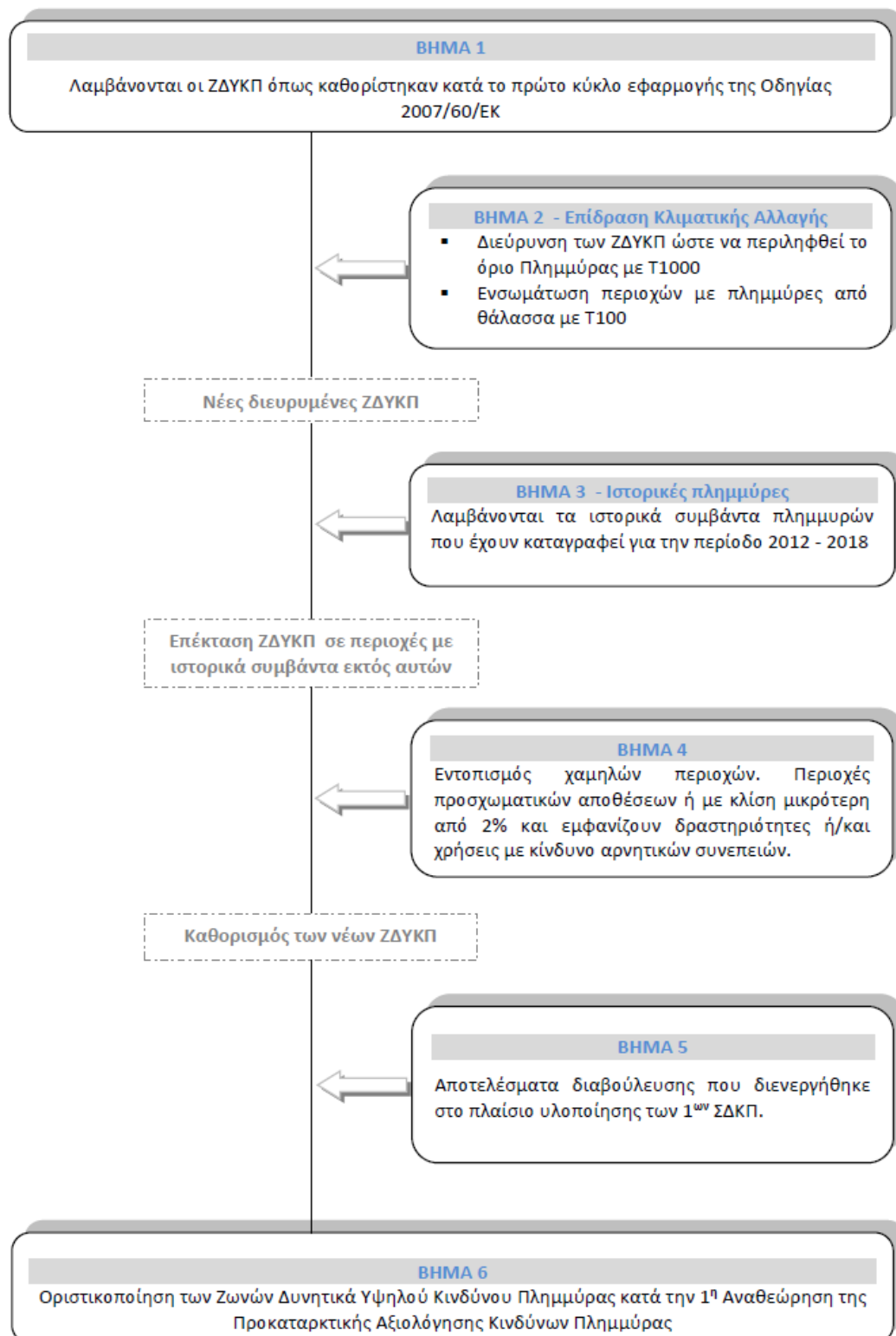
Σχήμα 4-2: Σχηματοποιημένη παρουσίαση της προσέγγισης αναθεώρησης των ΖΔΥΚΠ ΖΔΥΚΠ ΥΔ EL11
