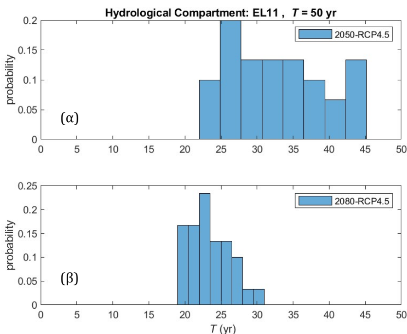
Σχήμα 4-12: Ποσοστά των σταθμών του ΥΔ EL11 ως συνάρτηση των νέων περιόδων επαναφοράς γεγονότων βροχής που, κατά την τρέχουσα περίοδο, αντιστοιχούν σε περίοδο επαναφοράς T = 50 έτη: α) μελλοντική περίοδος 2041-01-01 έως 2070-12-31 (2050s), και β) μελλοντική περίοδος 2071-01-01 έως 2100-12-31 (2080s).
