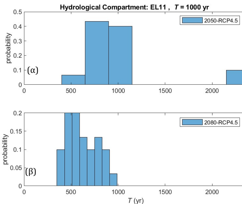
Σχήμα 4-14: Ποσοστά των σταθμών του ΥΔ EL11 ως συνάρτηση των νέων περιόδων επαναφοράς γεγονότων βροχής που, κατά την τρέχουσα περίοδο, αντιστοιχούν σε περίοδο επαναφοράς T = 1000 έτη: α) μελλοντική περίοδος 2041-01-01 έως 2070-12-31 (2050s), και β) μελλοντική περίοδος 2071-01-01 έως 2100-12-31 (2080s).
