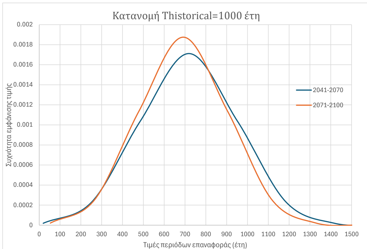
Εικόνα 2-17 Καμπύλη κατανομής Thistorical=1000 έτη
