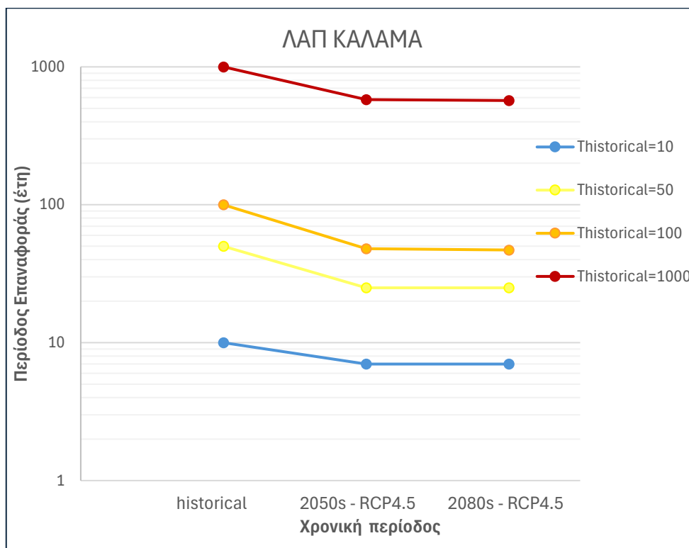
Εικόνα 2-10 Γράφημα επιρροής της κλιματική αλλαγής στη ΛΑΠ Καλαμά
