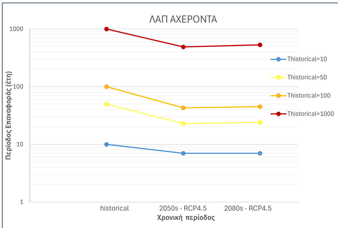
Εικόνα 2-14 Γράφημα επιρροής της κλιματική αλλαγής στη ΛΑΠ Αχέροντα
