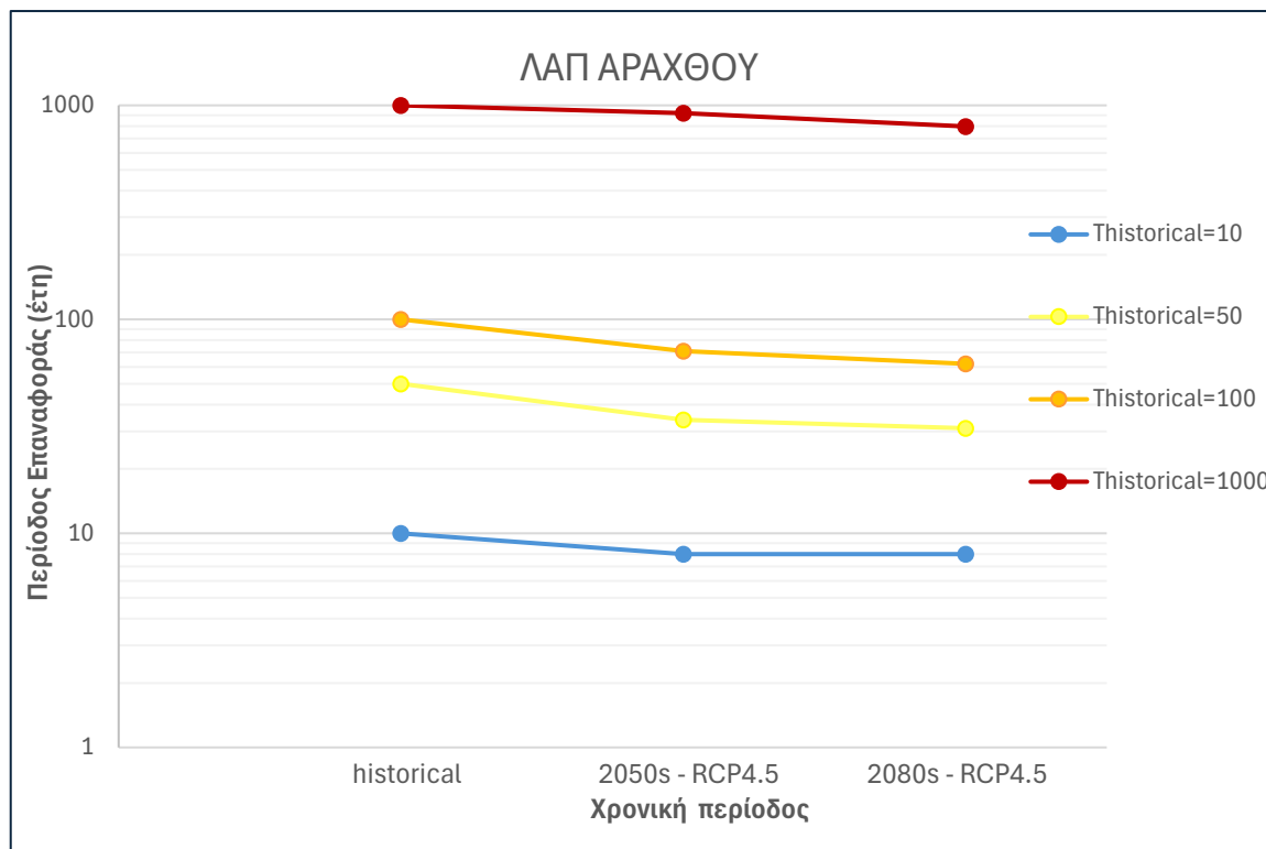
Εικόνα 2-12 Γράφημα επιρροής της κλιματική αλλαγής στη ΛΑΠ Αράχθου
