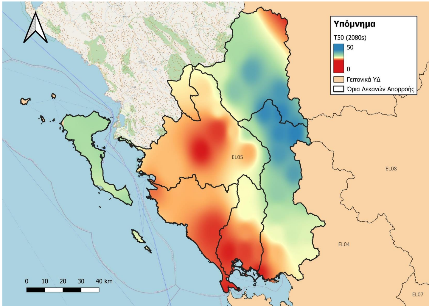
Εικόνα 2-5 Χάρτης Επιρροής της Κλιματικής Αλλαγής στην συχνότητα πλημμυρικών φαινομένων του ΥΔ05, με τρέχουσα περίοδο επαναφοράς T=50 έτη, κατά τη μελλοντική περίοδο 2071-2100
