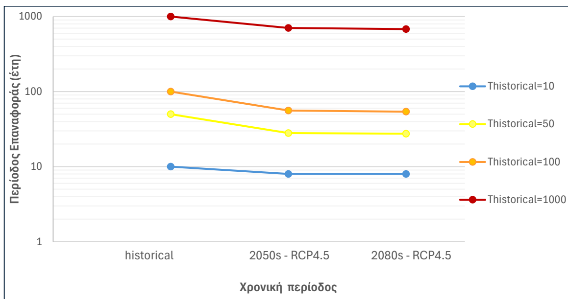
Εικόνα 2-3 Γράφημα επιρροής της κλιματική αλλαγής στο ΥΔ05
