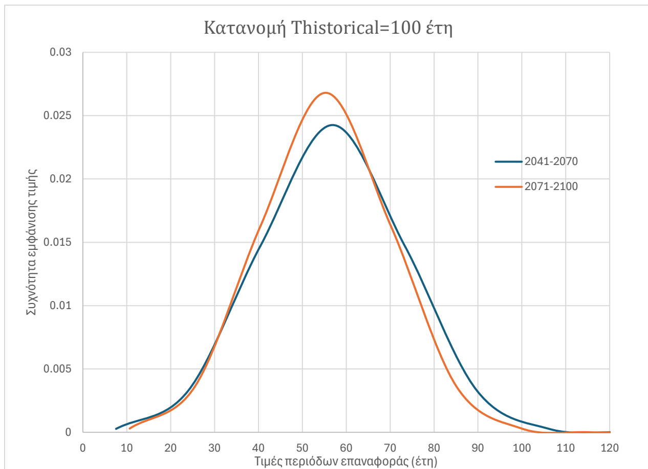
Εικόνα 2-16 Καμπύλη κατανομής Thistorical=100 έτη
