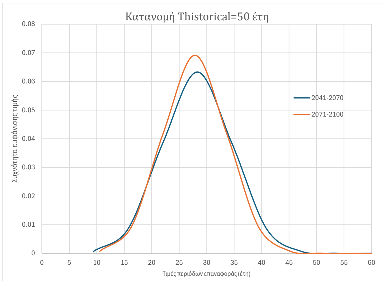
Εικόνα 2-15 Καμπύλη κατανομής Thistorical=50 έτη
