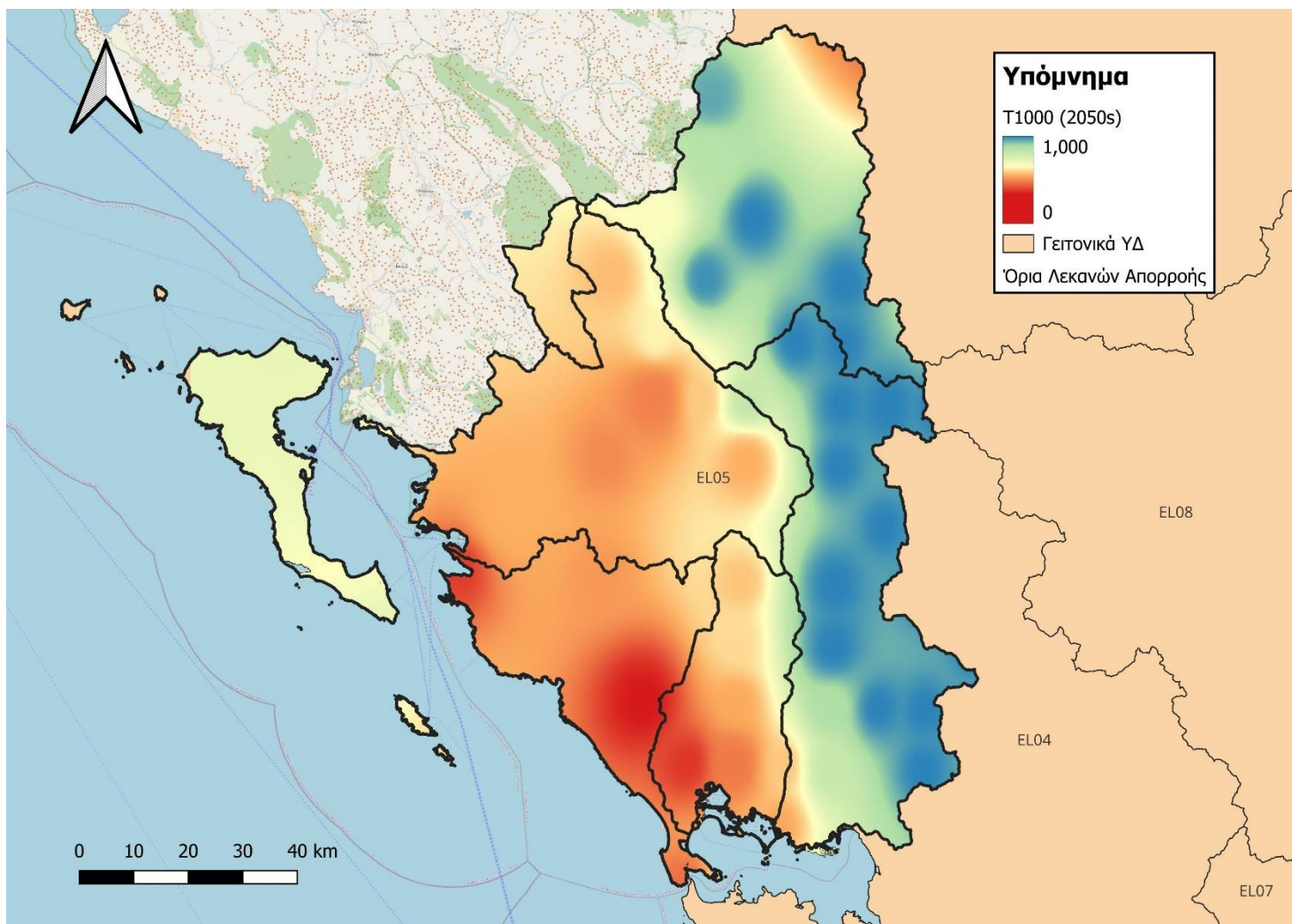
Εικόνα 2-8 Χάρτης Επιρροής της Κλιματικής Αλλαγής στην συχνότητα πλημμυρικών φαινομένων του ΥΔ05, με τρέχουσα περίοδο επαναφοράς T=1000 έτη, κατά τη μελλοντική περίοδο 2041-2070
