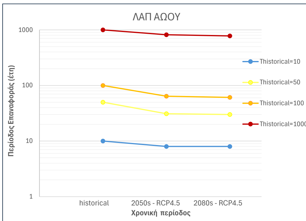
Εικόνα 2-11 Γράφημα επιρροής της κλιματικής αλλαγής στη ΛΑΠ Αώου
