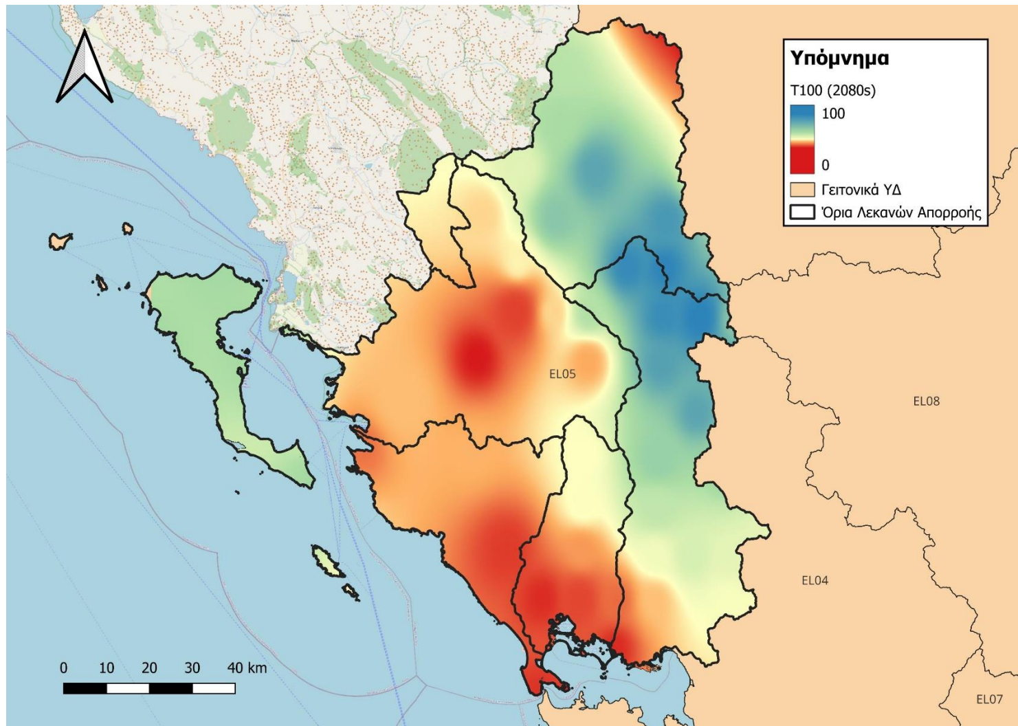
Εικόνα 2-7 Χάρτης Επιρροής της Κλιματικής Αλλαγής στην συχνότητα πλημμυρικών φαινομένων του ΥΔ05, με τρέχουσα περίοδο επαναφοράς T=100 έτη, κατά τη μελλοντική περίοδο 2071-2100
