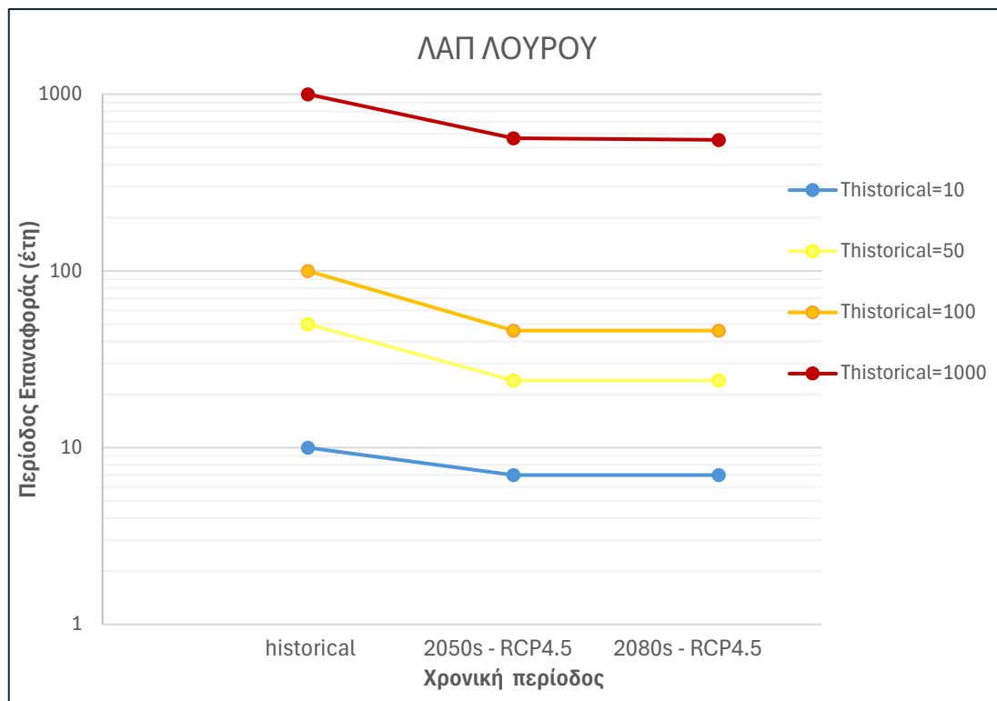
Εικόνα 2-13 Γράφημα επιρροής της κλιματικής αλλαγής στη ΛΑΠ Λούρου
