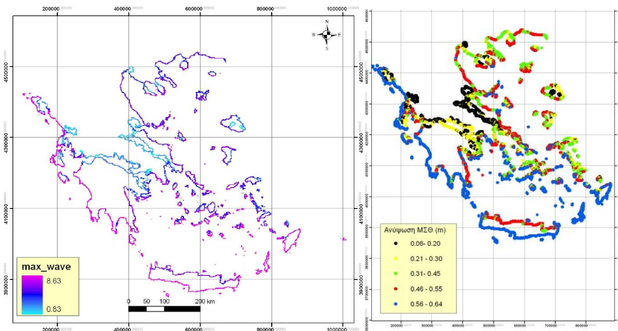
Σχήμα 4.11: Μέγιστο ύψος κύματος στην ακτογραμμή και μέγιστη ανύψωση ΜΣΘ από όλες τις διευθύνσεις
