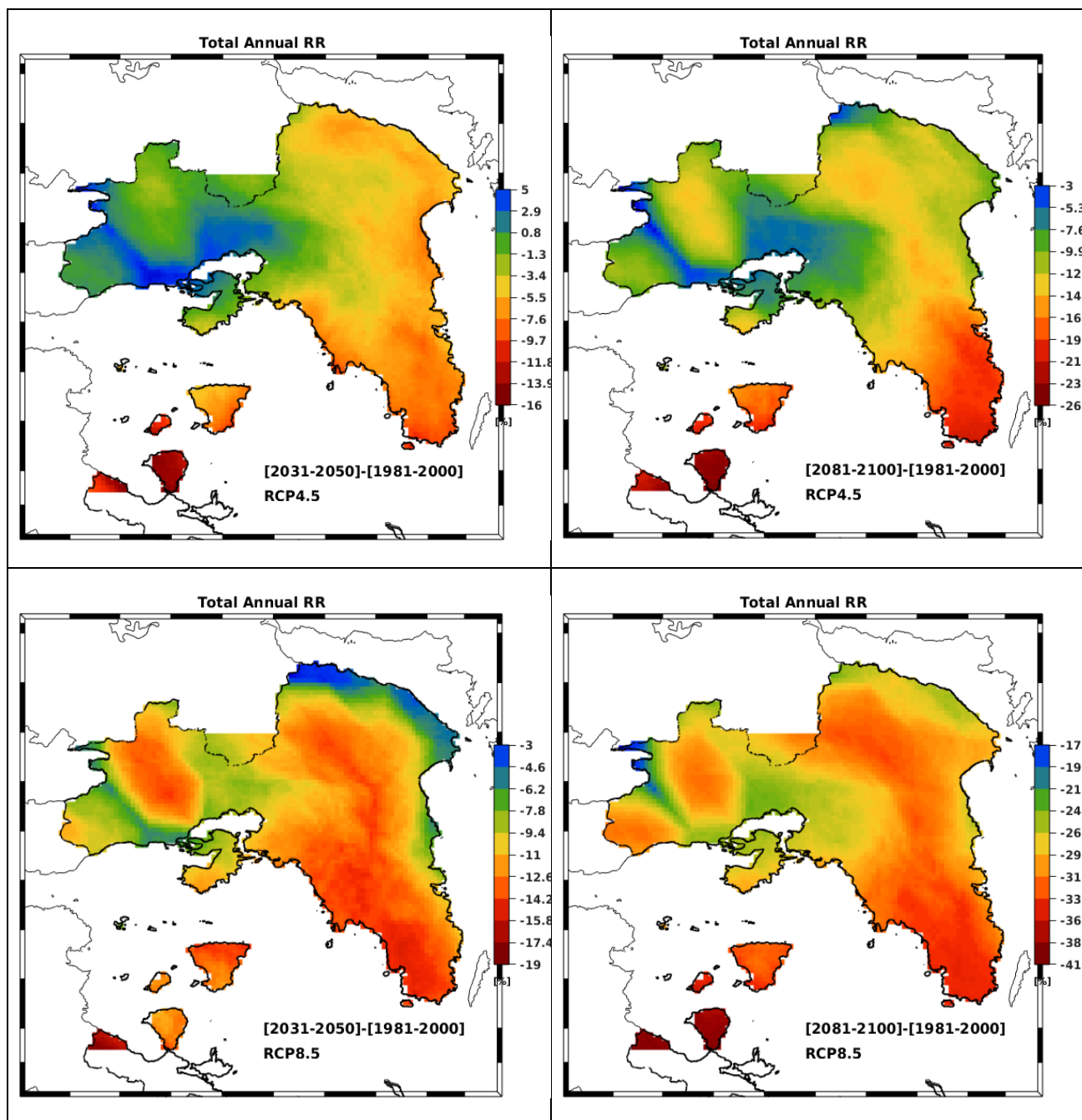
Σχήμα 3.8: Μεταβολή της συνολικής ετήσιας βροχόπτωσης για τις 2 μελλοντικές περιόδους 2031-2050 (αριστερά) και 2081-2100 (δεξιά) και για τα 2 κλιματικά σενάρια το RCP4.5 (επάνω) και το RCP8.5 (κάτω) σε σχέση με την περίοδο αναφοράς 1981-2000 στην Αττική
