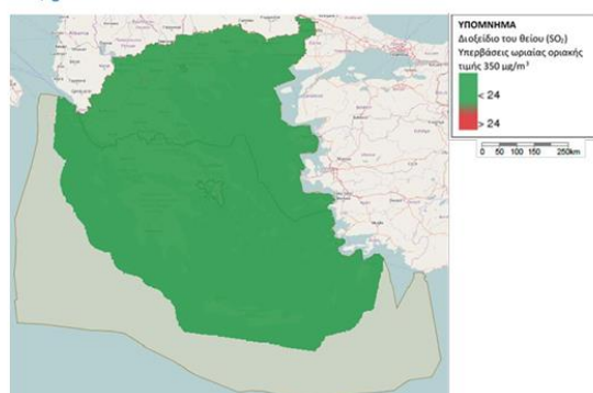
Διοξείδιο του θείου ( \text{SO}_2 ) - Υπερβάσεις ωριαίας οριακής τιμής 350 \mu\text{g}/\text{m}^3
