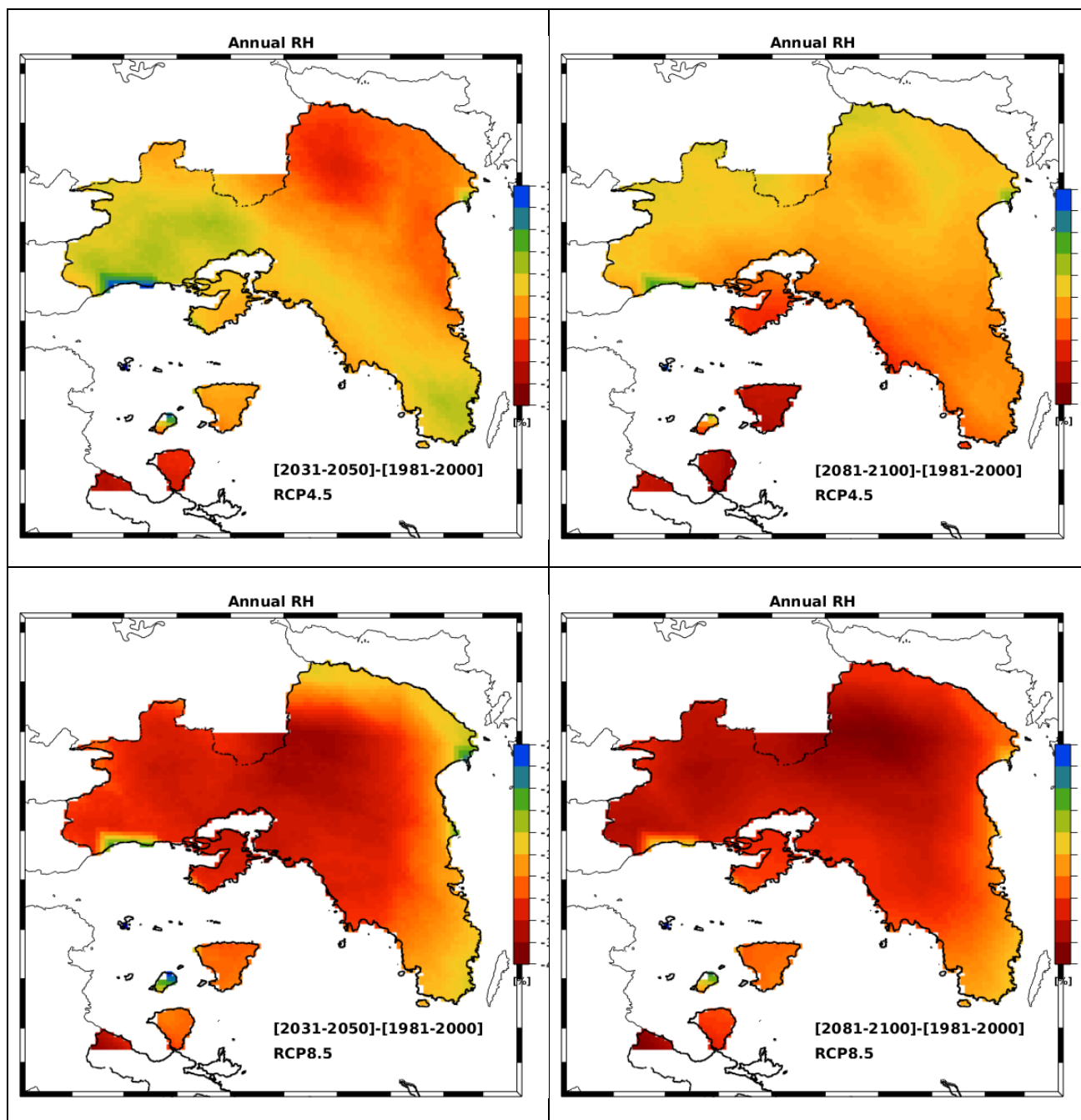
Σχήμα 3.9: Ποσοστιαίες μεταβολές της ετήσιας σχετικής υγρασίας για την Αττική σύμφωνα με τα σενάρια RCP4.5 (πάνω) και RCP8.5 (κάτω). Τα σχήματα αριστερά αφορούν μεταβολές μεταξύ του εγγύς μέλλοντος (2031-2050) και της περιόδου αναφοράς (1981-2000) και τα σχήματα δεξιά αφορούν μεταβολές μεταξύ του μακρινού μέλλοντος (2081-2100) και της περιόδου αναφοράς (1981-2000)
