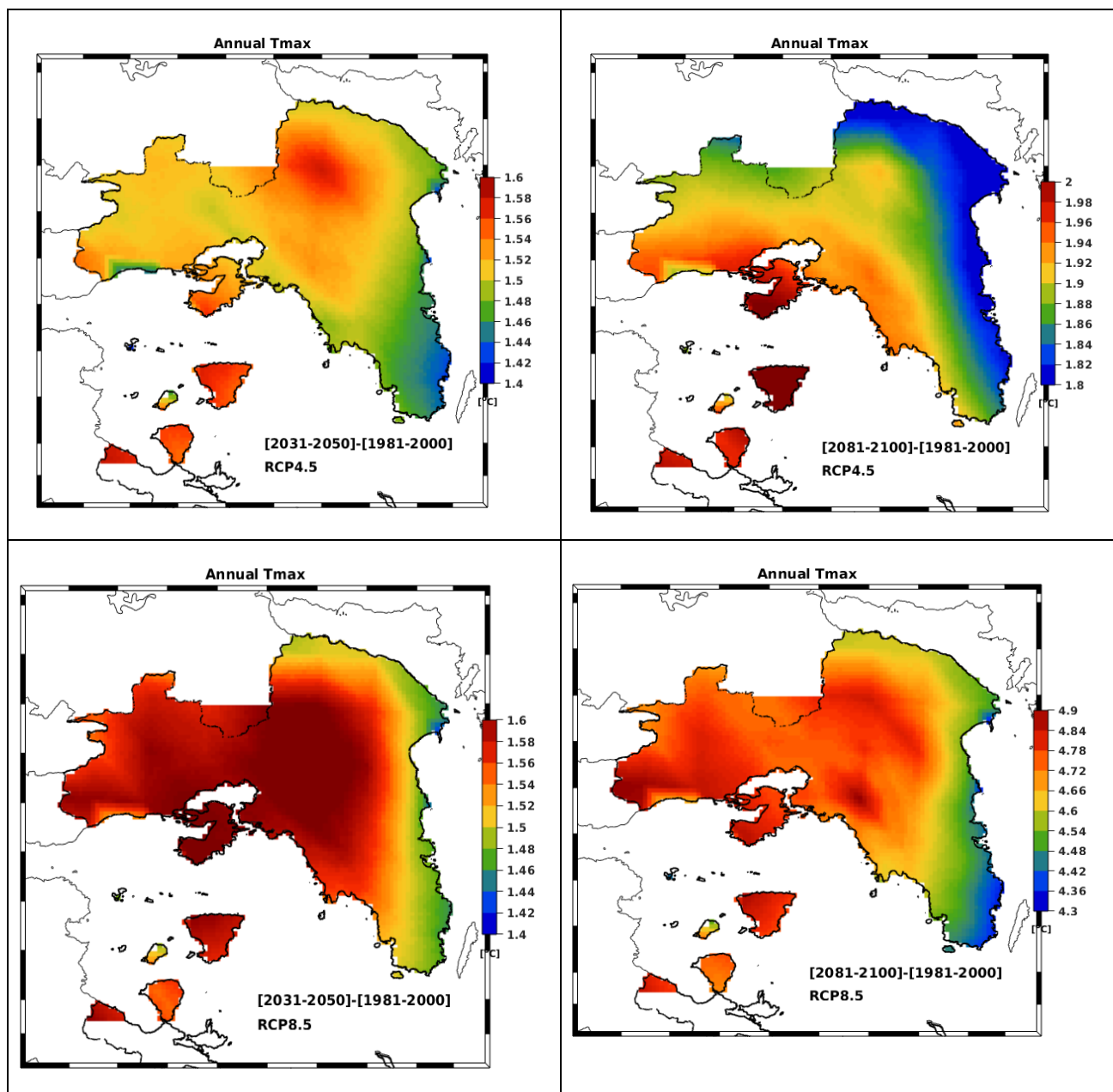
Σχήμα 3.7: Διαφορές των προβλέψεων της μέγιστης ετήσιας θερμοκρασίας για τις 2 μελλοντικές περιόδους 2031-2050 (αριστερά) και 2081-2100 (δεξιά) για τα 2 κλιματικά σενάρια το RCP4.5 (επάνω) και το RCP8.5 (κάτω) σε σχέση με τις αντίστοιχες θερμοκρασίες της περιόδου αναφοράς 1981-2000 για την Αττική
