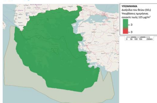
Διοξείδιο του θείου ( \text{SO}_2 ) - Υπερβάσεις ημερήσιας οριακής τιμής 125 \mu\text{g}/\text{m}^3
