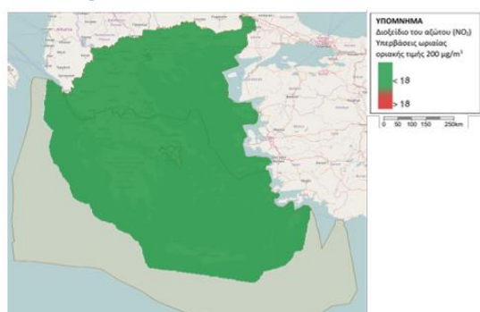
Διοξείδιο του αζώτου ( \text{NO}_2 ) - Υπερβάσεις ωριαίας οριακής τιμής 200 \mu\text{g}/\text{m}^3
