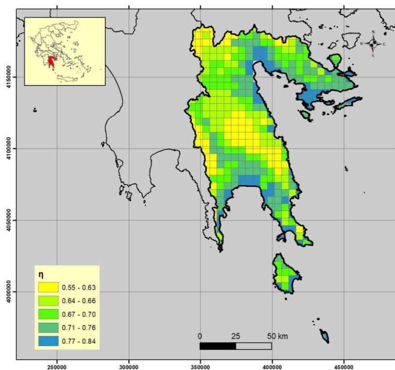
Σχήμα 4.14: Χωρική κατανομή παραμέτρου \eta^* για το ΥΔ Ανατολικής Πελοποννήσου (ΕΛ03)
