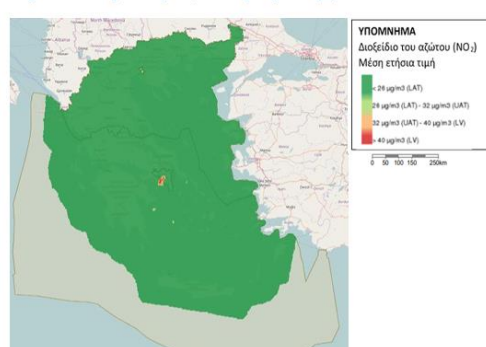
Διοξείδιο του αζώτου ( \text{NO}_2 ) - Μέση ετήσια τιμή
