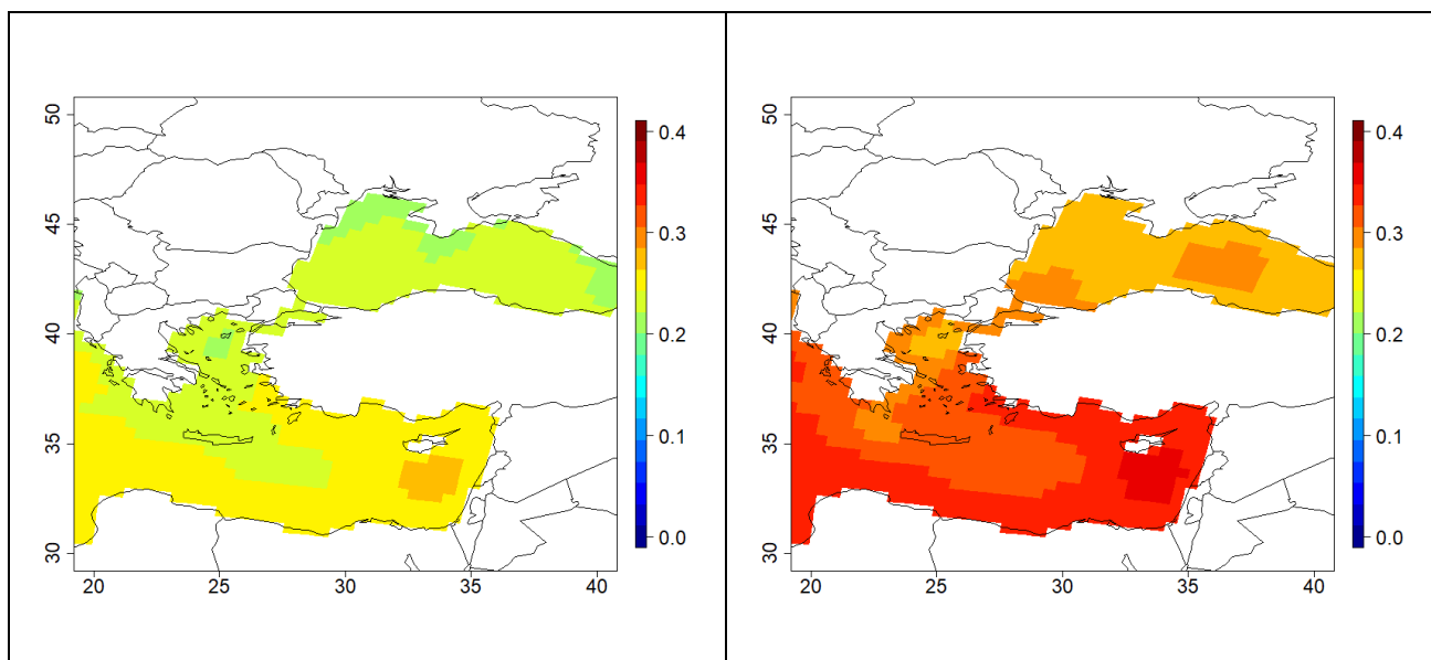
Σχήμα 3.12: Χωρική κατανομή της προβλεπόμενης μεταβολής της θαλάσσιας στάθμης για την περίοδο 2071-2100 (μακρινό μέλλον) σε σύγκριση με την περίοδο αναφοράς 1971-2000 για το σενάριο εκπομπών RCP4.5 (αριστερά) και το σενάριο εκπομπών RCP8.5 (δεξιά) με βάση το κλιματικό μοντέλο MPI-ESM-MR στην ανατολική Μεσόγειο
