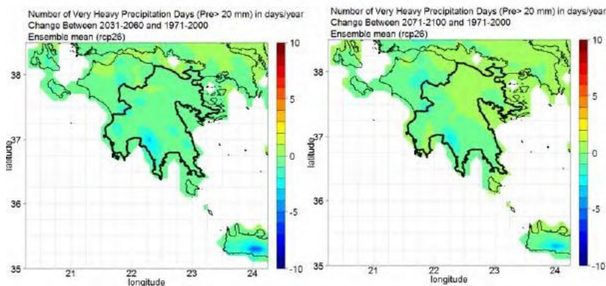
Σχήμα 3-17: Μεταβολές του αριθμού των ημερών με έντονη βροχόπτωση (>20mm, σε ημέρες/έτος) στην Περιφέρεια Πελοποννήσου σύμφωνα με τα σενάρια RCP2.6. Το αριστερό τμήμα αφορά μεταβολές μεταξύ
