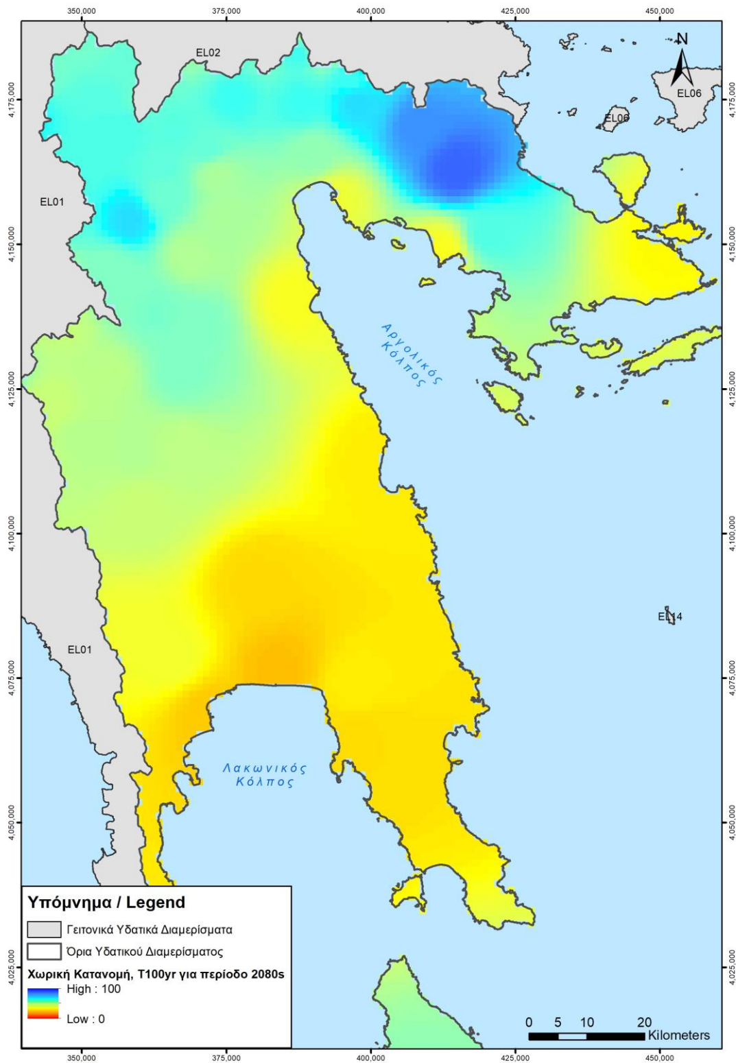
Σχήμα 2.8 : Χάρτης Επιρροής της Κλιματικής Αλλαγής στην συχνότητα πλημμυρικών φαινομένων του ΥΔ 03 με τρέχουσα περίοδο επαναφοράς T = 100 yrs, κατά την μελλοντική περίοδο 2071-2100.
