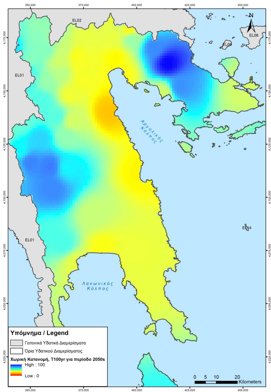
Σχήμα 2.7 : Χάρτης Επιρροής της Κλιματικής Αλλαγής στην συχνότητα πλημμυρικών φαινομένων του ΥΔ 03 με τρέχουσα περίοδο επαναφοράς T = 100 yrs, κατά την μελλοντική περίοδο 2041-2070.
