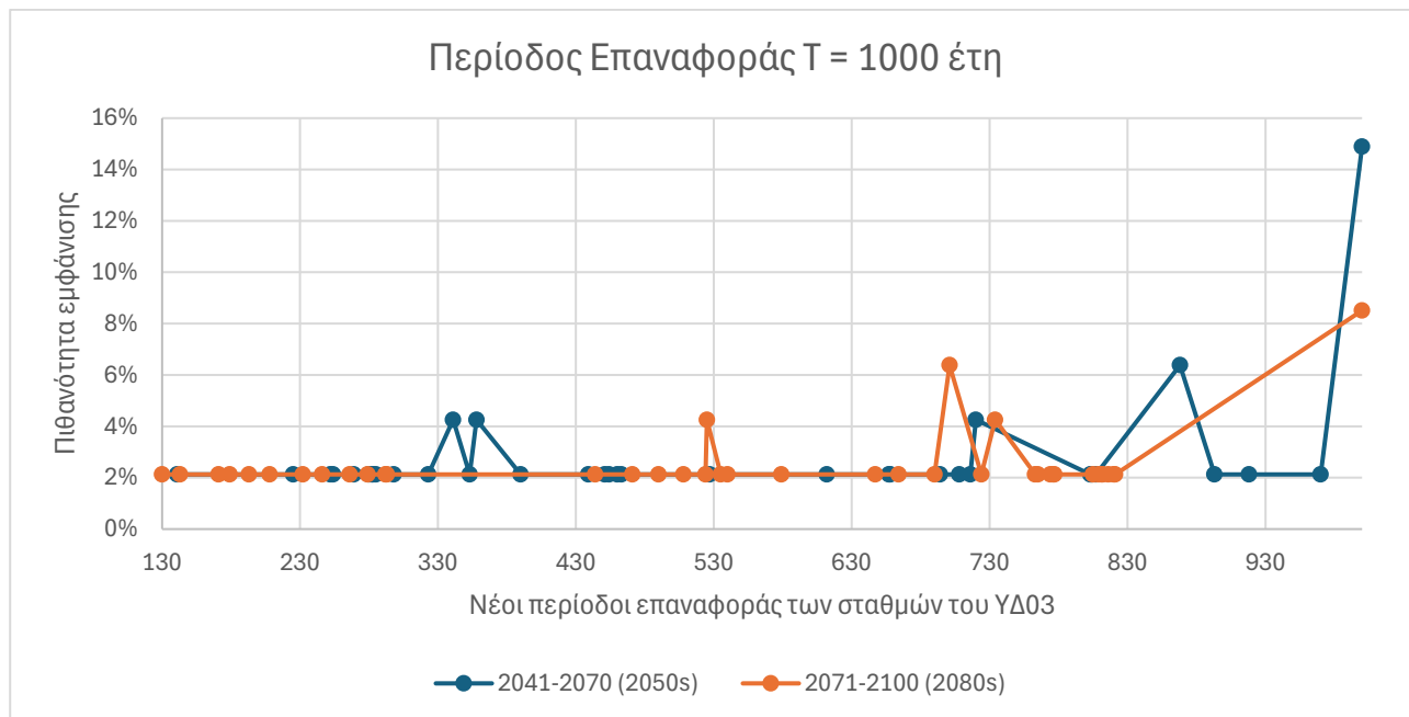
Σχήμα 2.17: Κατανομή των τιμών περιόδων επαναφοράς των σταθμών του ΥΔ 03 υπό κλιματική αλλαγή, για T=1000 σε κάθε μία από τις δύο μελλοντικές περιόδους που εξετάζονται.
