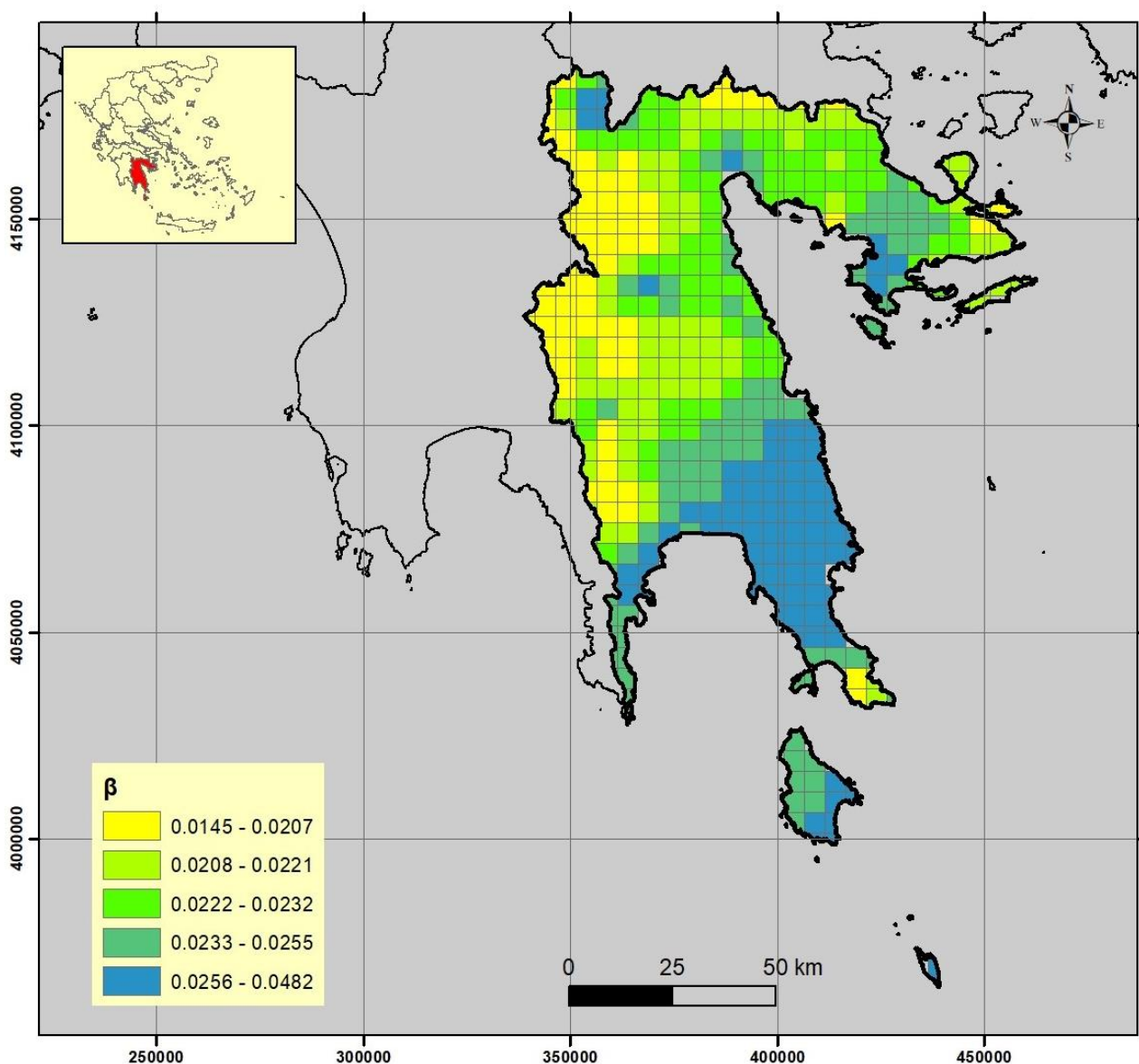
Σχήμα 2.3 : Χωρική κατανομή παραμέτρου «β» για το ΥΔ Ανατολικής Πελοποννήσου (EL03)
