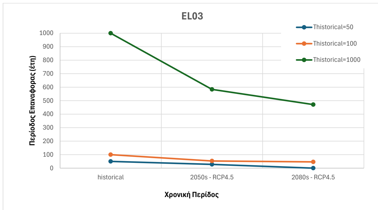
Σχήμα 2.11 : Επιρροή της κλιματικής αλλαγής στη συχνότητα εμφάνισης πλημμυρικών φαινομένων στο ΥΔ 03: μεταβολή της μέσης περιόδου επαναφοράς στο ΥΔ κατά τις μελλοντικές περιόδους 2041-2070 και 2071 - 2100.
