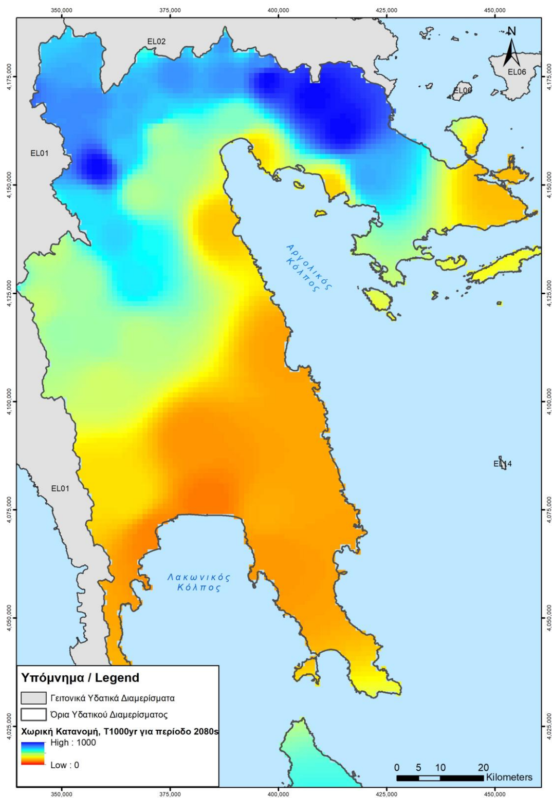
Σχήμα 2.10 : Χάρτης Επιρροής της Κλιματικής Αλλαγής στην συχνότητα πλημμυρικών φαινομένων του ΥΔ 03 με τρέχουσα περίοδο επαναφοράς T = 1000 yrs, κατά την μελλοντική περίοδο 2071-2100.
