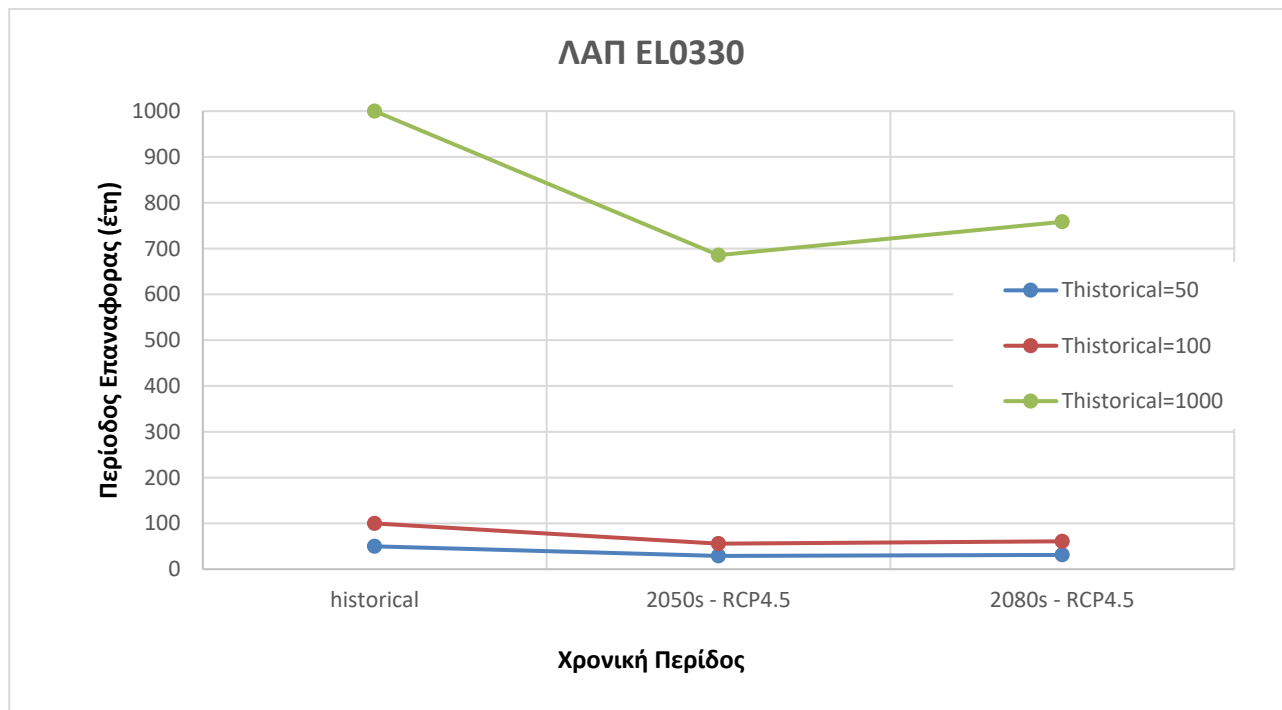
Σχήμα 2.14 : Επιρροή της κλιματικής αλλαγής στη συχνότητα εμφάνισης πλημμυρικών φαινομένων στη ΛΑΠ EL30 του ΥΔ 03: μεταβολή της μέσης περιόδου επαναφοράς στο ΥΔ κατά τις μελλοντικές περιόδους 2041-2070 και 2071 - 2100.
