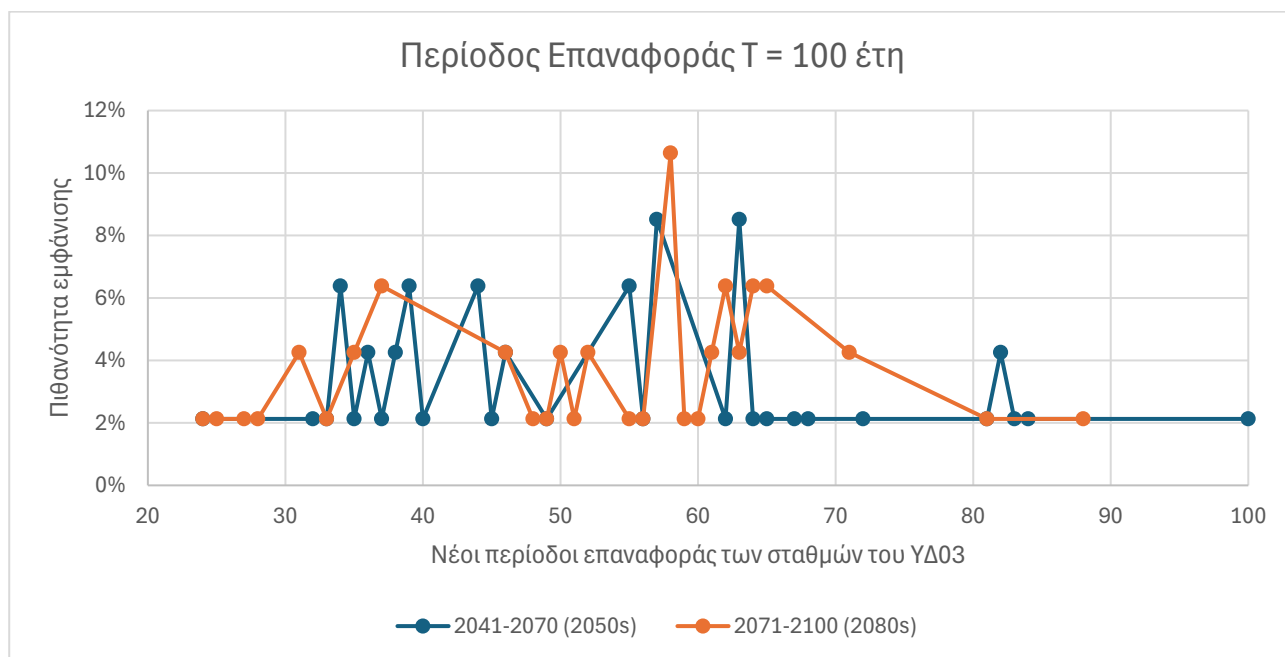
Σχήμα 2.16: Κατανομή των τιμών περιόδων επαναφοράς των σταθμών του ΥΔ 03 υπό κλιματική αλλαγή, για T=100 σε κάθε μία από τις δύο μελλοντικές περιόδους που εξετάζονται.
