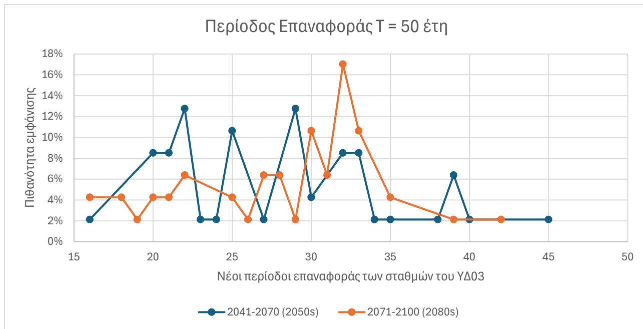
Σχήμα 2.15: Κατανομή των τιμών περιόδων επαναφοράς των σταθμών του ΥΔ 03 υπό κλιματική αλλαγή, για T=50 σε κάθε μία από τις δύο μελλοντικές περιόδους που εξετάζονται.
