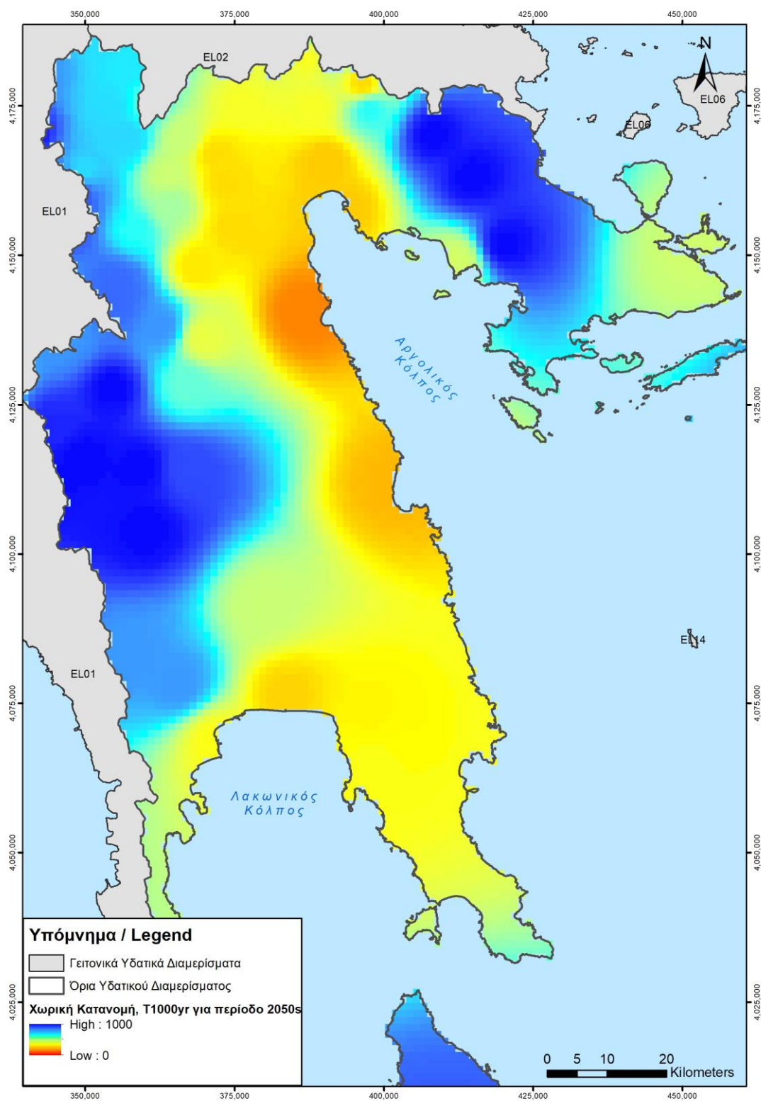
Σχήμα 2.9 : Χάρτης Επιρροής της Κλιματικής Αλλαγής στην συχνότητα πλημμυρικών φαινομένων του ΥΔ 03 με τρέχουσα περίοδο επαναφοράς T = 1000 yrs, κατά την μελλοντική περίοδο 2041-2070.
