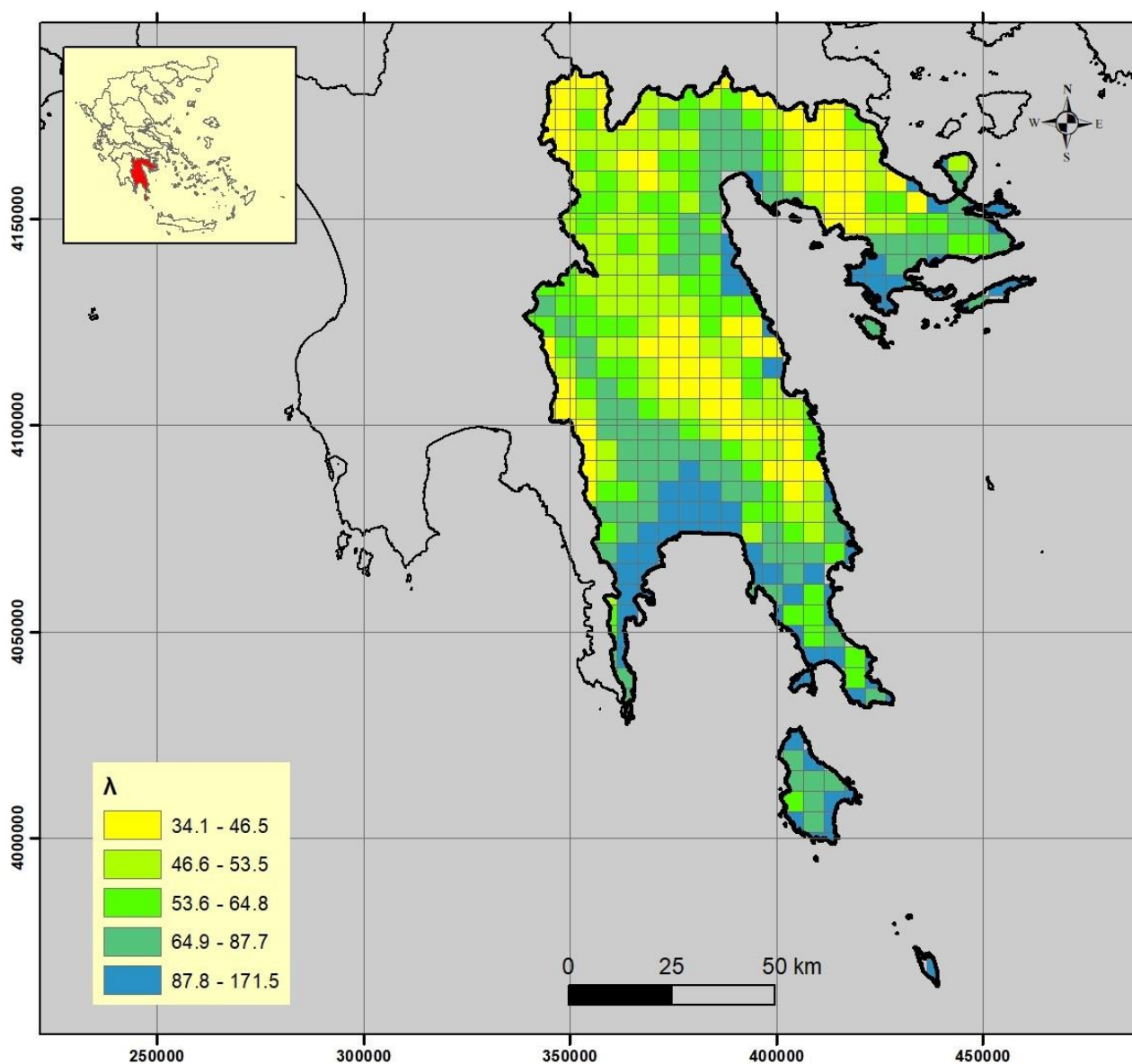
Σχήμα 2.4 : Χωρική κατανομή παραμέτρου «λ» για το ΥΔ Ανατολικής Πελοποννήσου (ΕΛ03)
