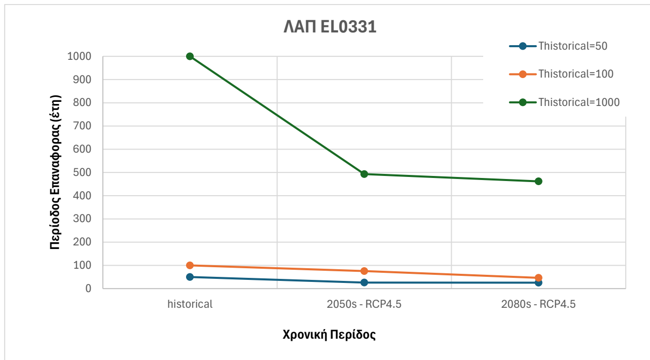
Σχήμα 2.12 : Επιρροή της κλιματικής αλλαγής στη συχνότητα εμφάνισης πλημμυρικών φαινομένων στη ΛΑΠ ΕΛ31 του ΥΔ 03: μεταβολή της μέσης περιόδου επαναφοράς στο ΥΔ κατά τις μελλοντικές περιόδους 2041-2070 και 2071 - 2100.
