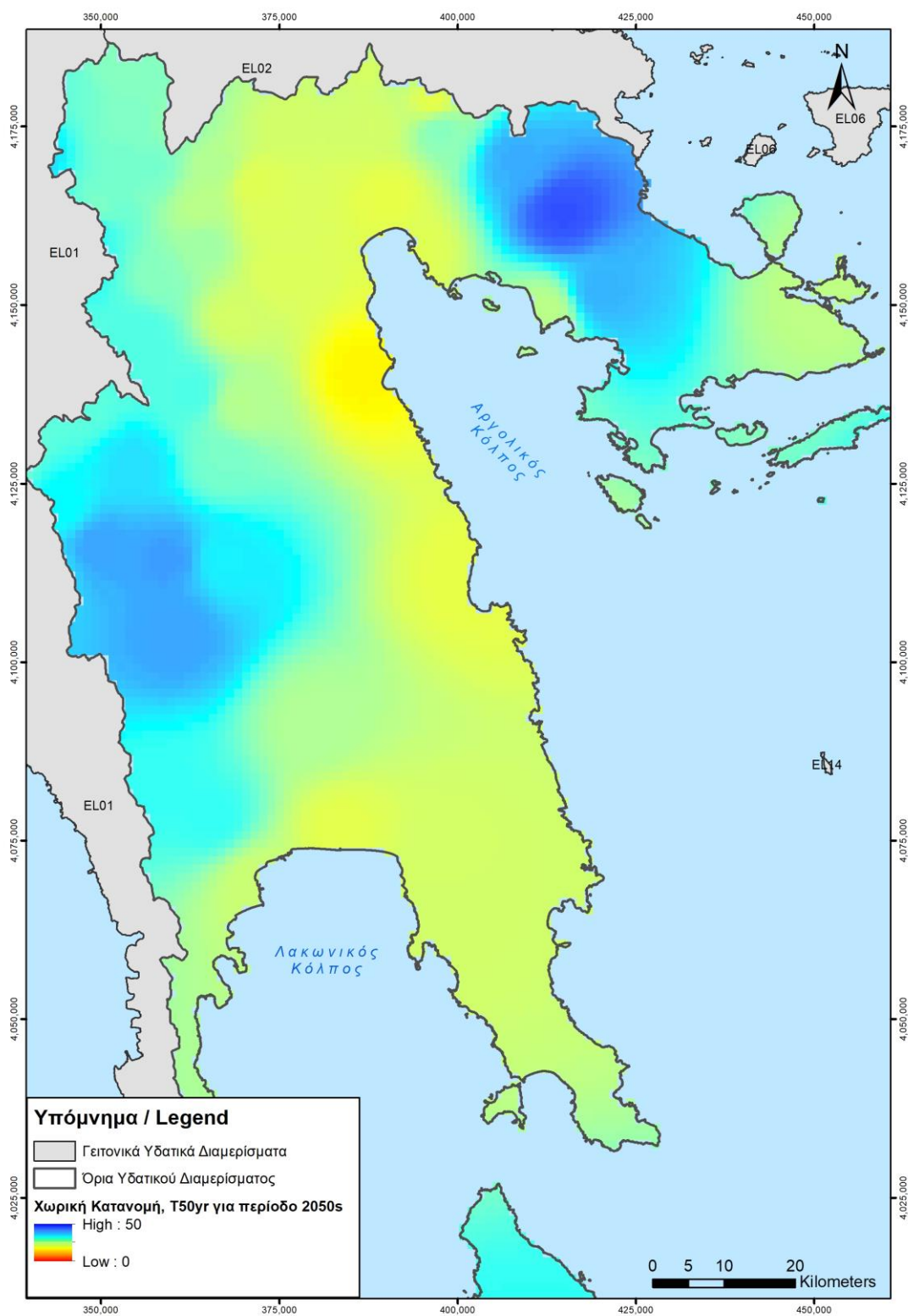
Σχήμα 2.5 : Χάρτης Επιρροής της Κλιματικής Αλλαγής στην συχνότητα πλημμυρικών φαινομένων του ΥΔ 03 με τρέχουσα περίοδο επαναφοράς T = 50 yrs, κατά την μελλοντική περίοδο 2041-2070.
