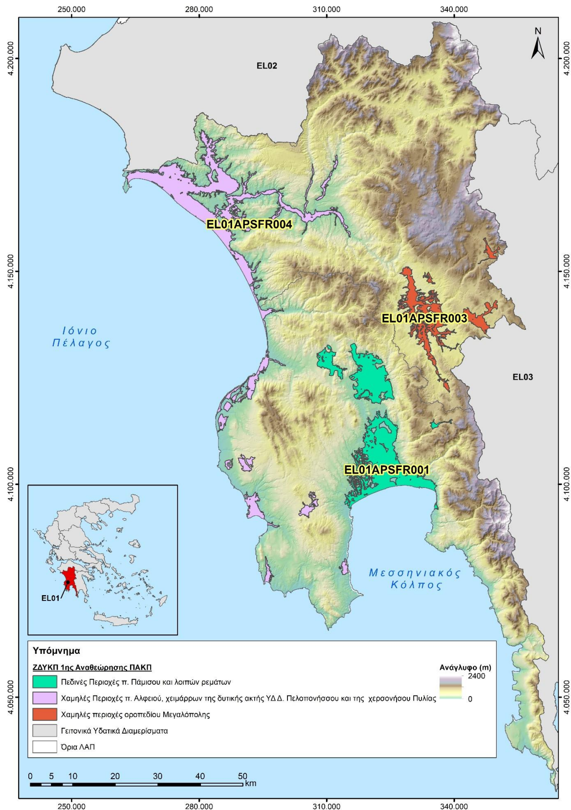
Σχήμα 3.1 : Ζώνες Δυνητικά Υψηλού Κινδύνου Πλημμύρας της 1ης Αναθεώρησης της ΠΑΚΠ για το ΥΔ Δυτικής Πελοποννήσου
