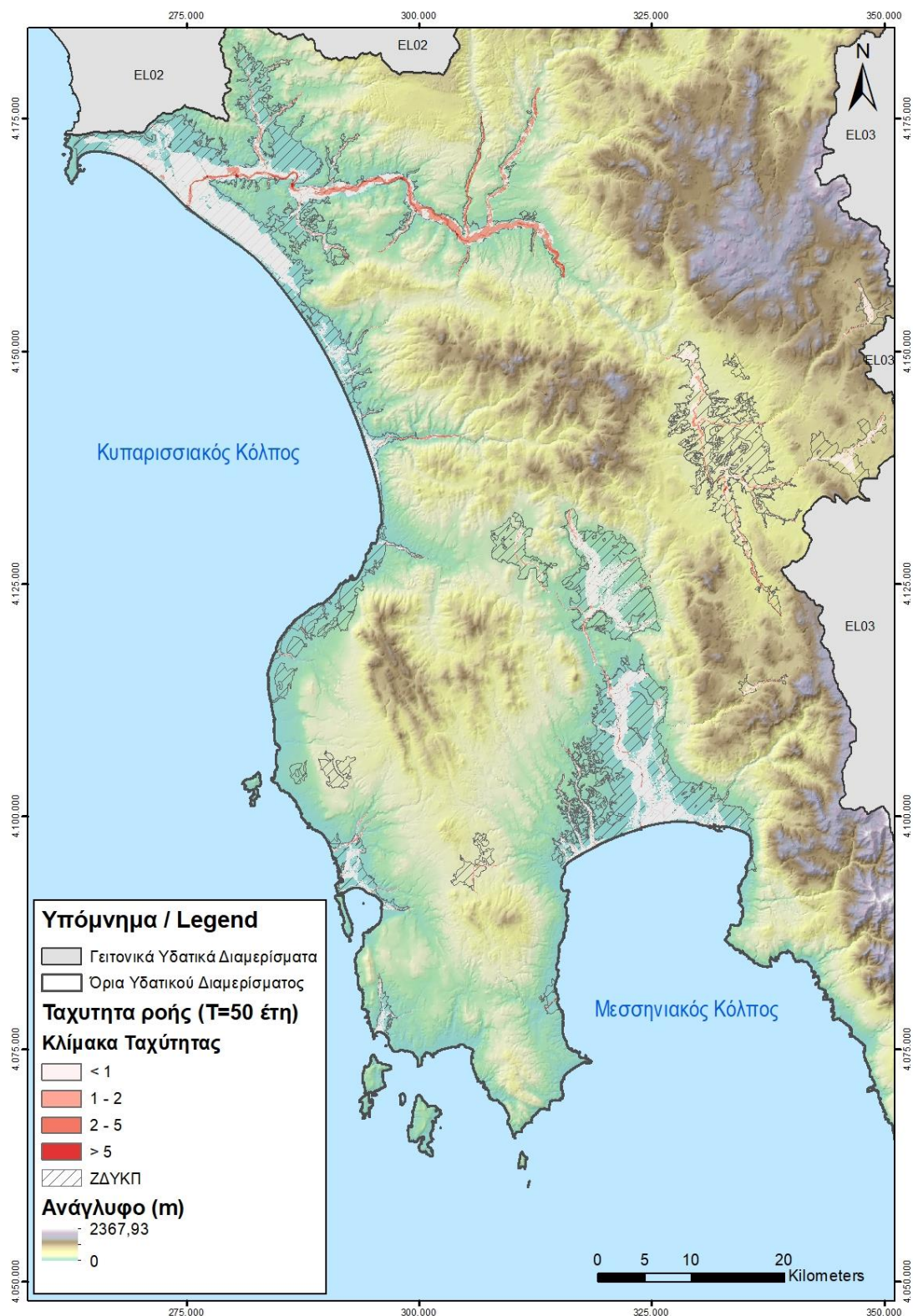
Σχήμα 4.4 : Ταχύτητα ροής για πλημμύρα με περίοδο επαναφοράς T=50 έτη για το Υδατικό Διαμέρισμα της Δυτικής Πελοποννήσου (EL01)
