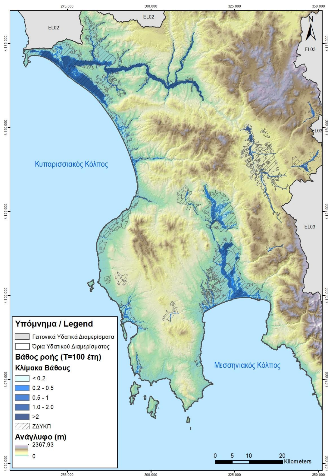
Σχήμα 4.2 : Βάθος ροής και μέγιστο εύρος κατάληψης για πλημμύρα με περίοδο επαναφοράς T=100 έτη για το Υδατικό Διαμέρισμα της Δυτικής Πελοποννήσου (EL01)
