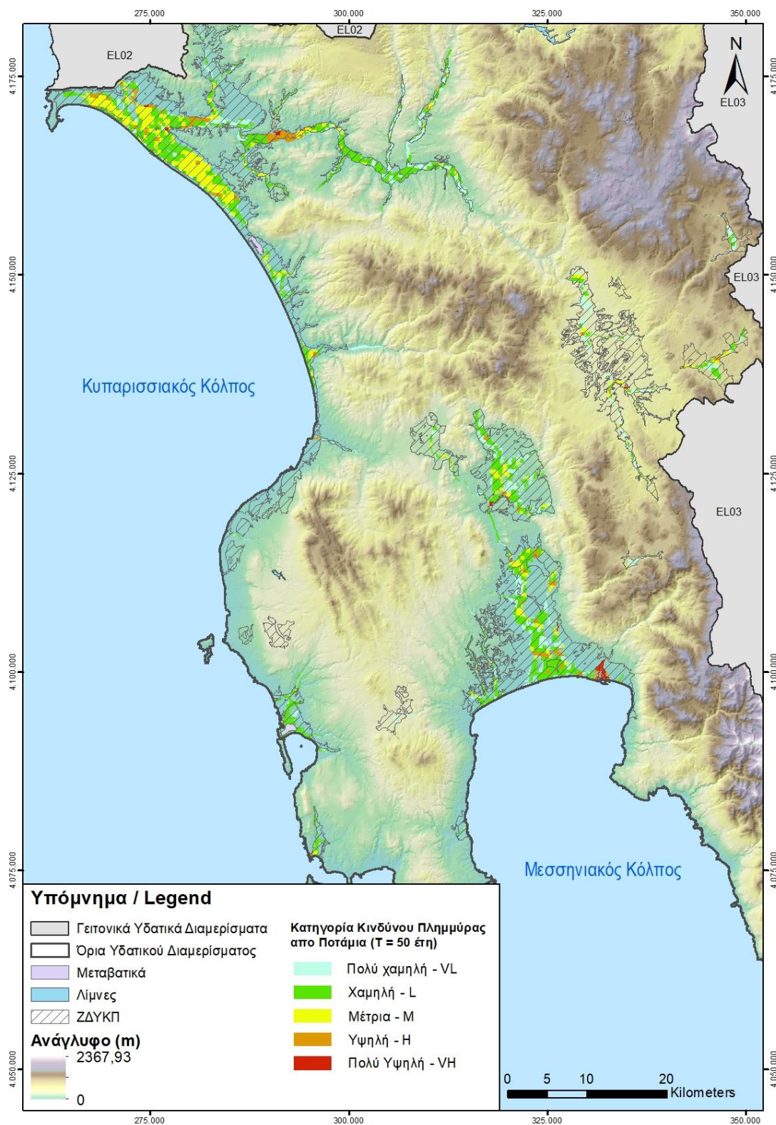
Σχήμα 5.2: Συνολική χωρική αξιολόγηση πλημμυρικού κινδύνου (Flood Risk) για T=50 έτη - EL01
