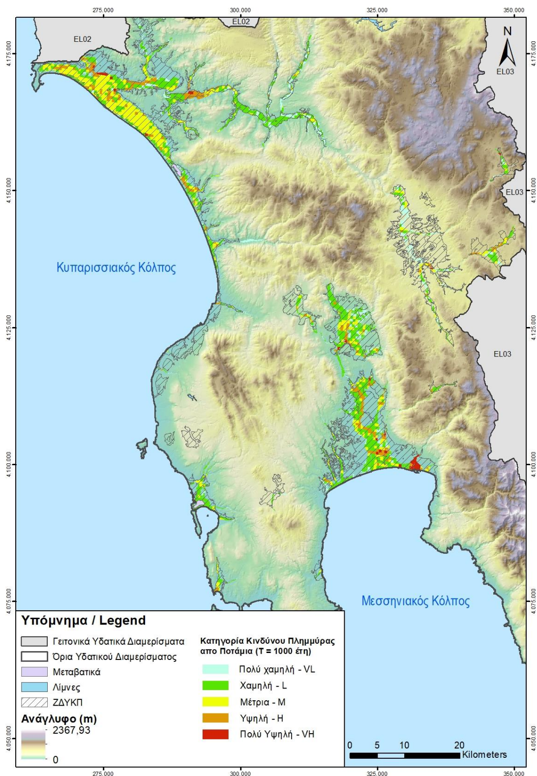
Σχήμα 5.4: Συνολική χωρική αξιολόγηση πλημμυρικού κινδύνου (Flood Risk) για T=1000 έτη - EL01
