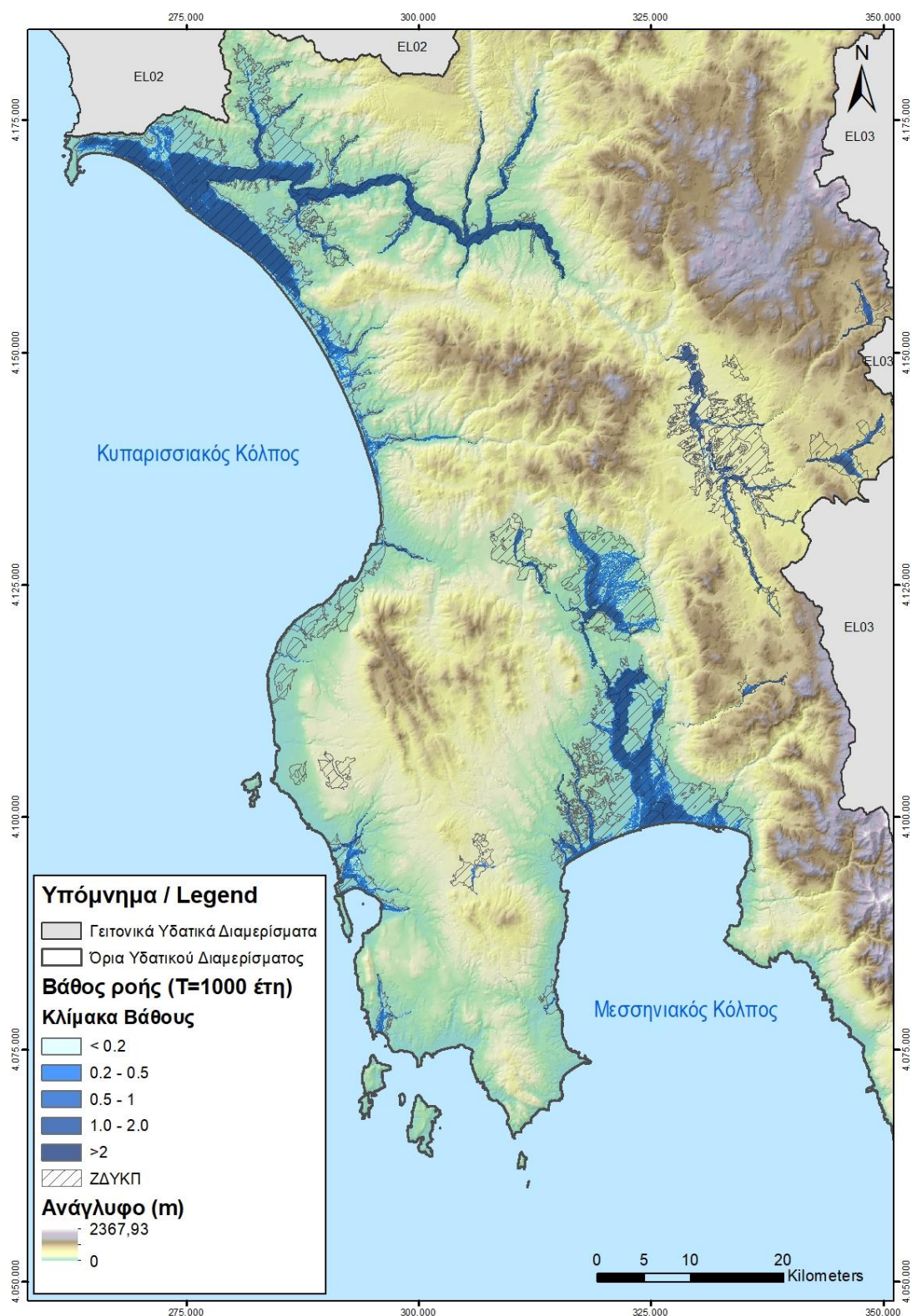
Σχήμα 4.3 : Βάθος ροής και μέγιστο εύρος κατάληψης για πλημμύρα με περίοδο επαναφοράς T=1000 έτη για το Υδατικό Διαμέρισμα της Δυτικής Πελοποννήσου (EL01)
