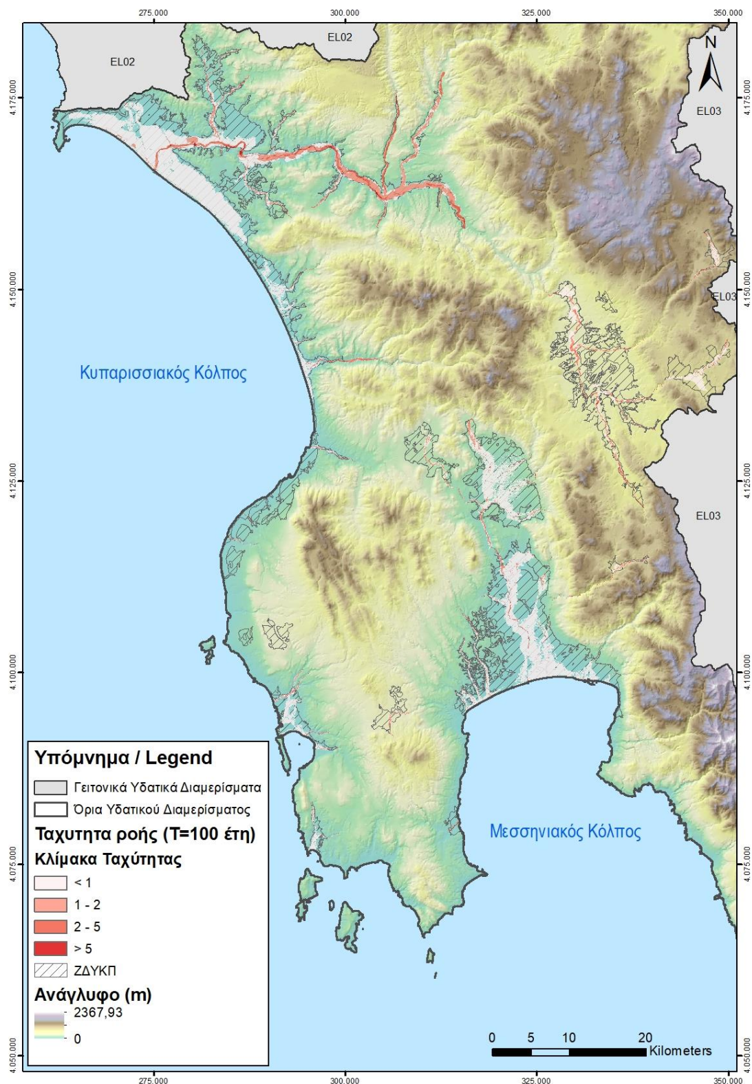
Σχήμα 4.5 : Ταχύτητα ροής για πλημμύρα με περίοδο επαναφοράς T=100 έτη για το Υδατικό Διαμέρισμα της Δυτικής Πελοποννήσου (EL01)
