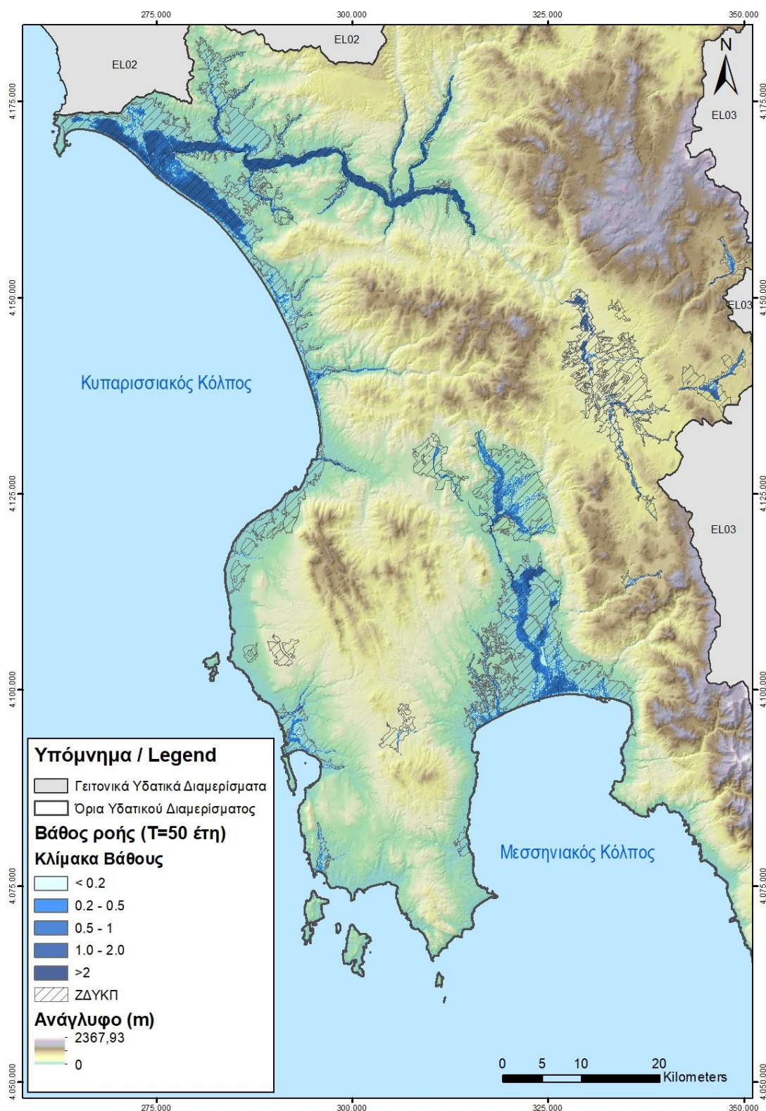
Σχήμα 4.1 : Βάθος ροής και μέγιστο εύρος κατάληψης για πλημμύρα με περίοδο επαναφοράς T=50 έτη για το Υδατικό Διαμέρισμα της Δυτικής Πελοποννήσου (EL01)
