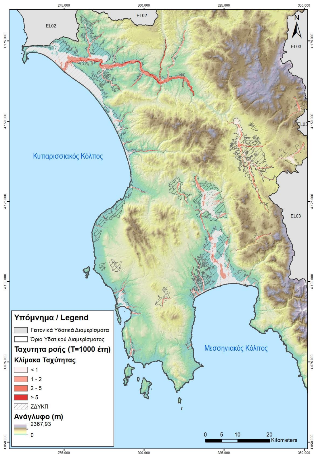
Σχήμα 4.6 : Ταχύτητα ροής για πλημμύρα με περίοδο επαναφοράς T=1000 έτη για το Υδατικό Διαμέρισμα της Δυτικής Πελοποννήσου (EL01)
