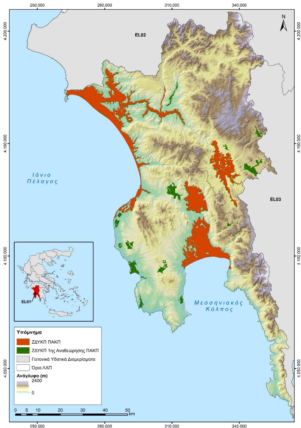
Σχήμα 2.4: Ζώνες Δυσνητικά υψηλού Κινδύνου Πλημμύρας της ΠΑΚΠ (κόκκινο) και της 1ης Αναθεώρησης της ΠΑΚΠ (πράσινο) στο ΥΔ Δυτικής Πελοποννήσου (EL01)
