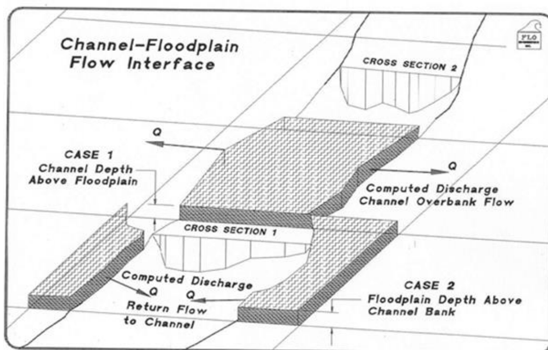
Σχήμα 3.11: Κίνηση ροής μεταξύ καναλιού και πεδιάδας
