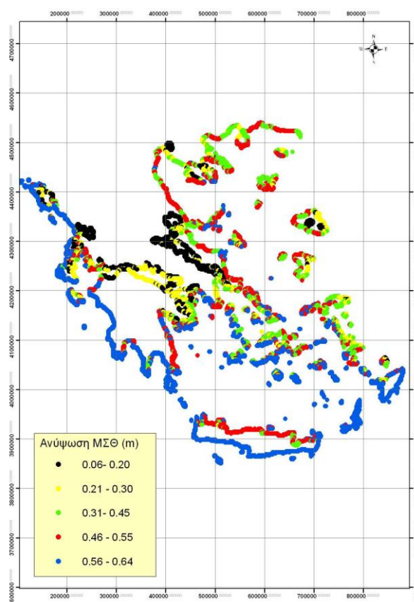
Σχήμα 3.5: Μέγιστη ανύψωση ΜΣΘ στην ακτογραμμή από κυματισμό
