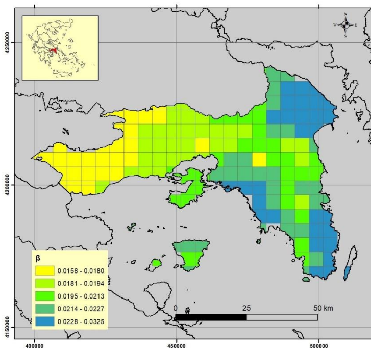
Σχήμα 3.8: Γεωγραφική κατανομή παραμέτρου \beta .
