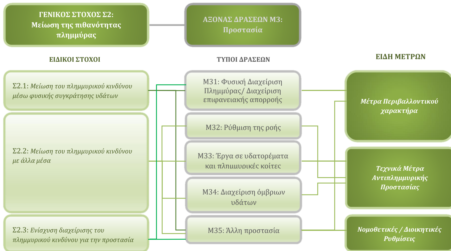
Εικόνα 4-3: Διάγραμμα συσχέτισης Γενικού Στόχου Σ2 - Ειδικών Στόχων με Τύπους Δράσεων και Είδη Μέτρων 1 ης Αναθεώρησης ΣΔΚΠ του Άξονα Μ3 Προστασία (οι διαφορετικοί χρωματισμοί των γραμμών έχουν ως αποκλειστικό σκοπό την ευκρίνεια του διαγράμματος)
