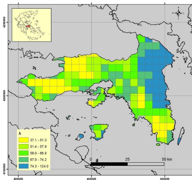
Σχήμα 3.9: Γεωγραφική κατανομή παραμέτρου λ.
