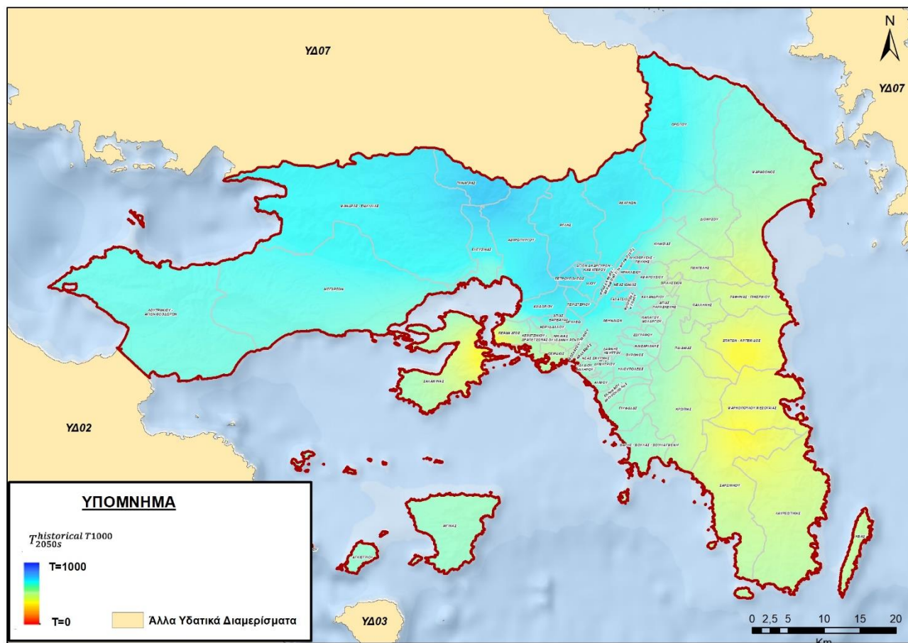
Σχήμα 3.32: Χάρτης χωρικής κατανομής των νέων περιόδων επαναφοράς T_{historical} T_{1000}^{2050s} για την κλιματική περίοδο 2041-2070 (2050s) των γεγονότων βροχής που κατά την τρέχουσα περίοδο αντιστοιχούν σε περιόδους επαναφοράς T=1000 έτη
