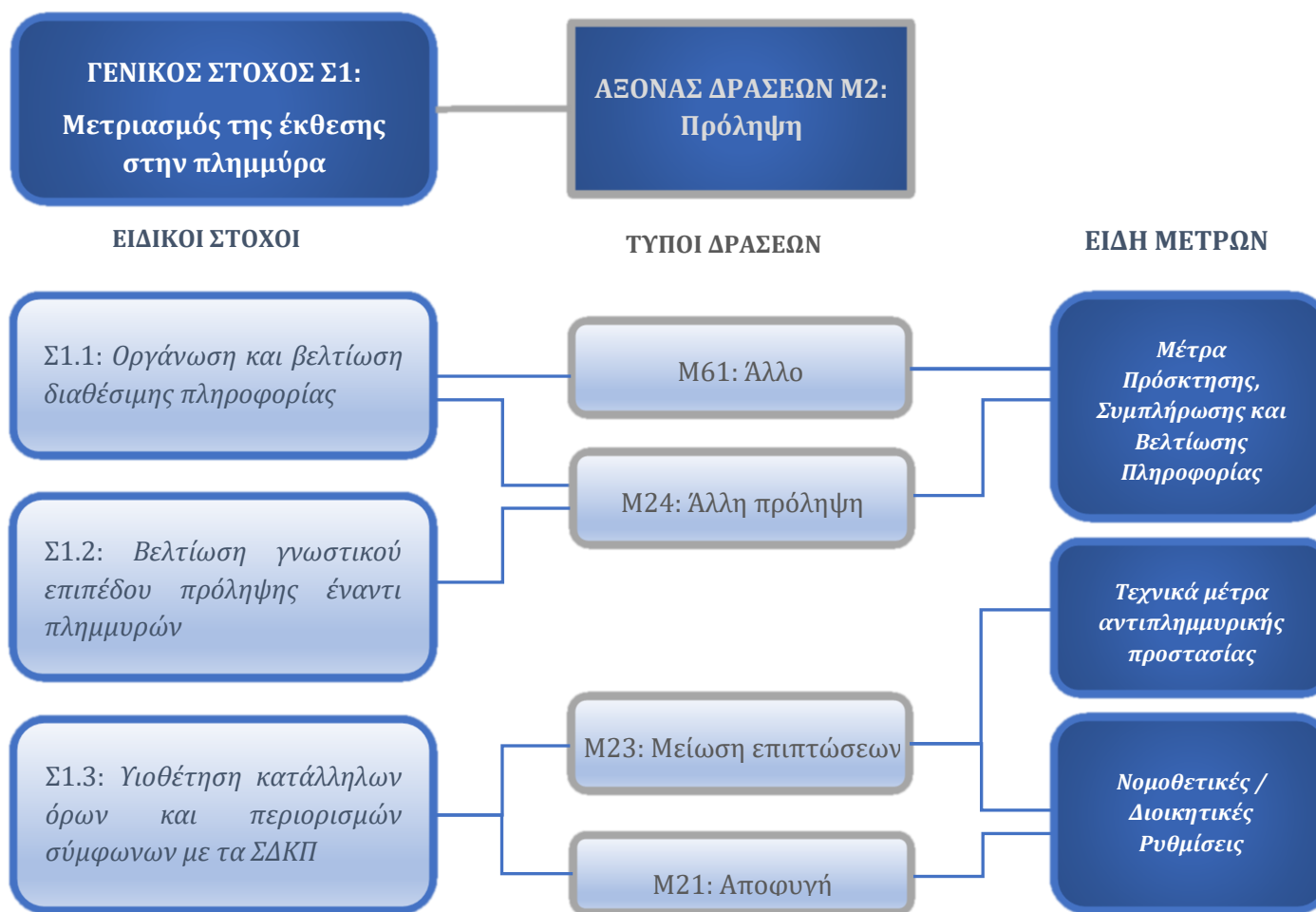
Εικόνα 4-2: Διάγραμμα συσχέτισης Γενικού Στόχου Σ1 - Ειδικών Στόχων με Τύπους Δράσεων και Είδη Μέτρων 1 ης Αναθεώρησης ΣΔΚΠ του Άξονα M2 Πρόληψη
