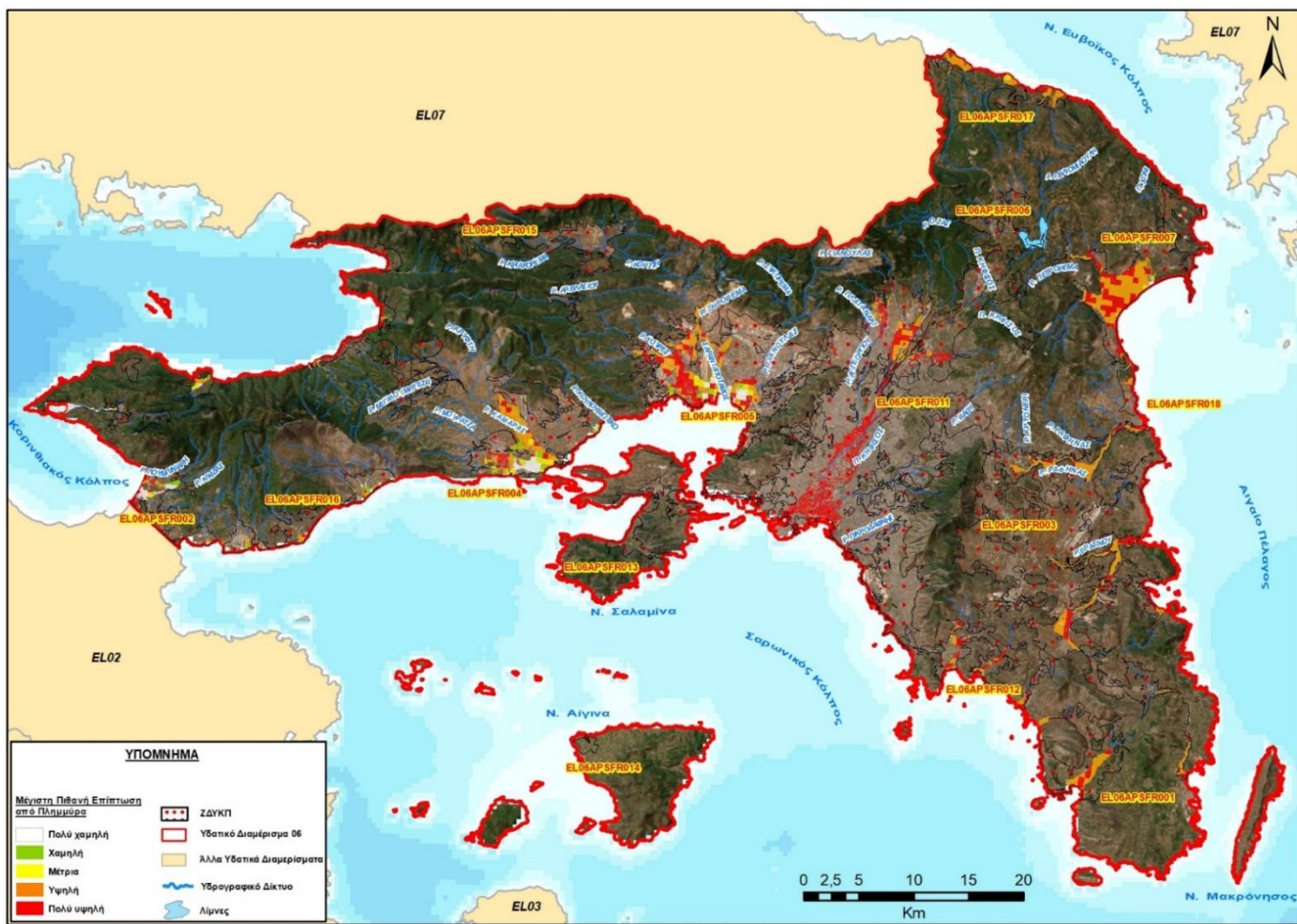
Σχήμα 3.22:Χάρτης μέγιστης πιθανής επίπτωσης πλημμύρας ΥΔ Αττικής (EL06) (T=1000 έτη)
