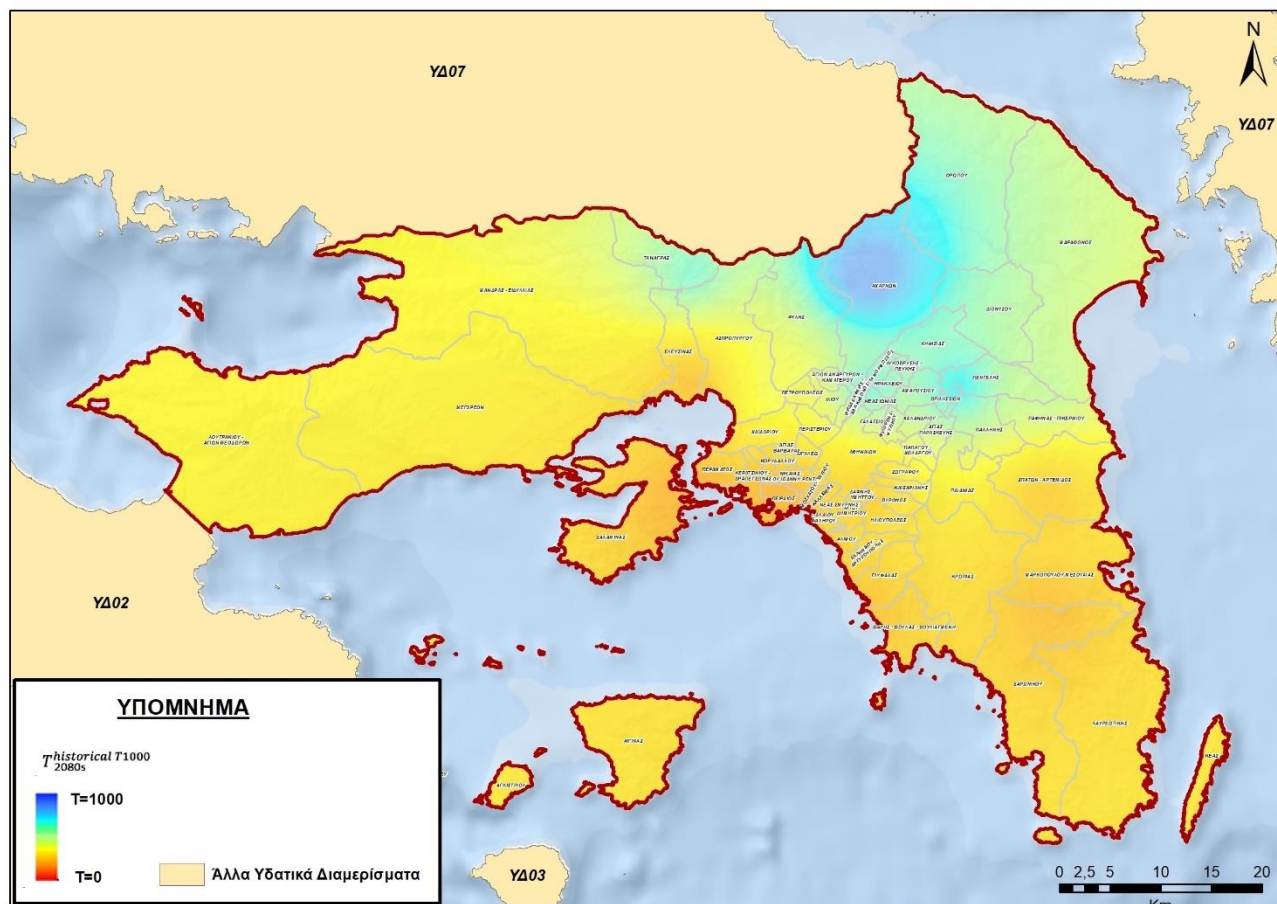
Σχήμα 3.35: Χάρτης χωρικής κατανομής των νέων περιόδων επαναφοράς T_{historical T1000 2080s} για την κλιματική περίοδο 2071-2100 (2080s) των γεγονότων βροχής που κατά την τρέχουσα περίοδο αντιστοιχούν σε περιόδους επαναφοράς T=1000 έτη
