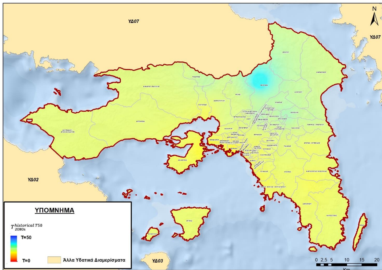
Σχήμα 3.33: Χάρτης χωρικής κατανομής των νέων περιόδων επαναφοράς T_{historical T50}^{2080s} για την κλιματική περίοδο 2071-2100 (2080s) των γεγονότων βροχής που κατά την τρέχουσα περίοδο αντιστοιχούν σε περιόδους επαναφοράς T=50 έτη
