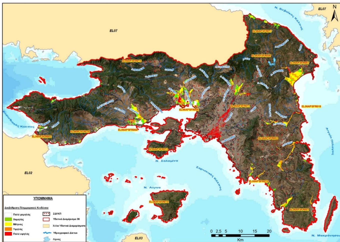
Σχήμα 3.28: Χάρτης αποτίμησης επιπτώσεων πλημμύρας ΥΔ Αττικής (EL06) (T=1000 έτη)
