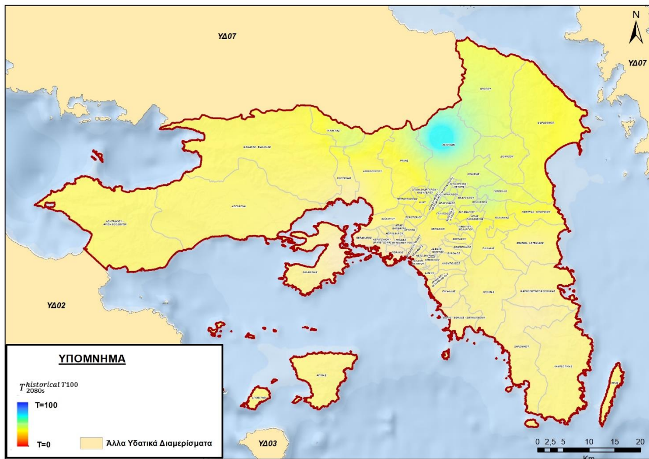
Σχήμα 3.34: Χάρτης χωρικής κατανομής των νέων περιόδων επαναφοράς T_{historical}^{T100} για την κλιματική περίοδο 2071-2100 (2080s) των γεγονότων βροχής που κατά την τρέχουσα περίοδο αντιστοιχούν σε περιόδους επαναφοράς T=100 έτη
