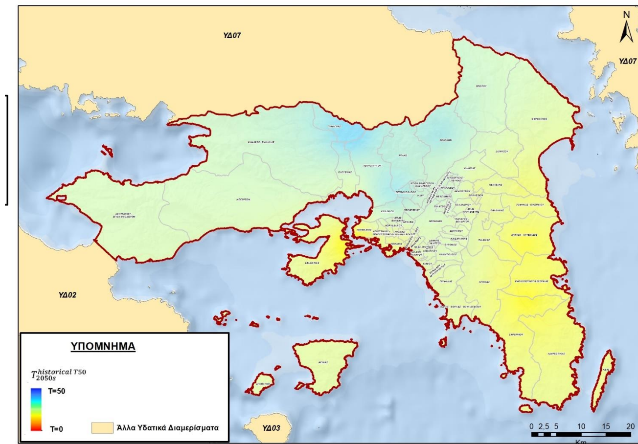
Σχήμα 3.30: Χάρτης χωρικής κατανομής των νέων περιόδων επαναφοράς T_{2050s}^{historical T50} για την κλιματική περίοδο 2041-2070 (2050s) των γεγονότων βροχής που κατά την τρέχουσα περίοδο αντιστοιχούν σε περιόδους επαναφοράς T=50 έτη
