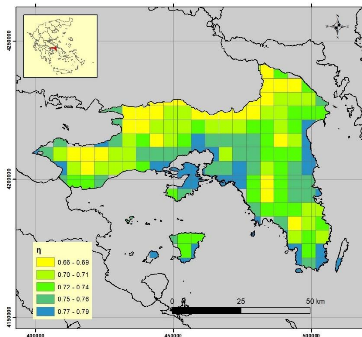
Σχήμα 3.7: Γεωγραφική κατανομή παραμέτρου \eta .
