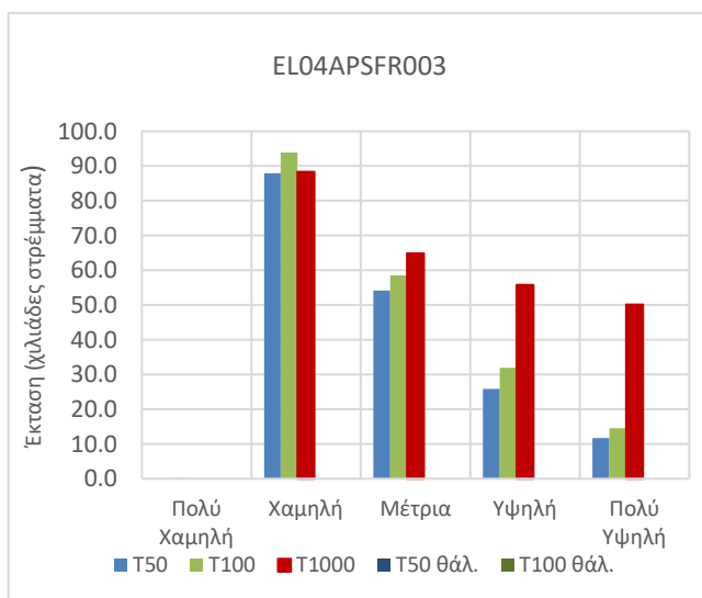
Εικόνα 3-74 Έκταση που αντιστοιχεί σε κάθε κατηγορία επικινδυνότητας πλημμύρας, ανά περίοδο επαναφοράς για τη EL04APSR003
