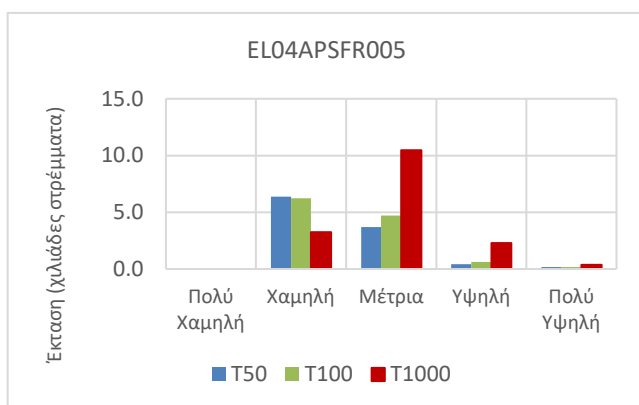
Εικόνα 3-80 Έκταση που αντιστοιχεί σε κάθε κατηγορία επικινδυνότητας πλημμύρας, ανά περίοδο επαναφοράς για τη EL04APSFR005
