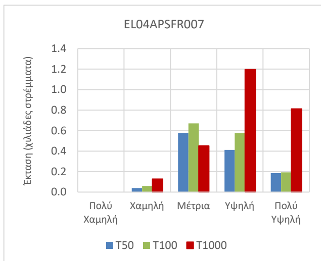
Εικόνα 3-86 Έκταση που αντιστοιχεί σε κάθε κατηγορία επικινδυνότητας πλημμύρας, ανά περίοδο επαναφοράς για τη EL04APSFR007
