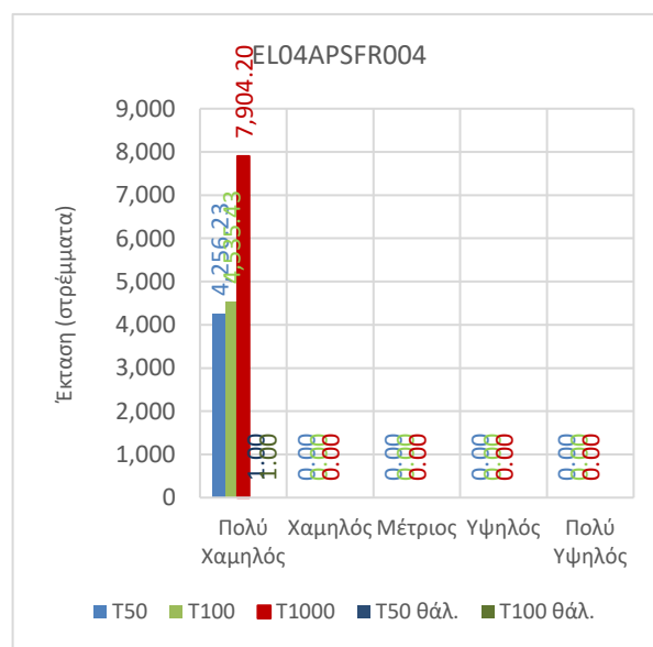
Εικόνα 3-78 Έκταση που αντιστοιχεί σε κάθε κατηγορία κινδύνου πλημμύρας, ανά περίοδο επαναφοράς για τη EL04APSFR004
