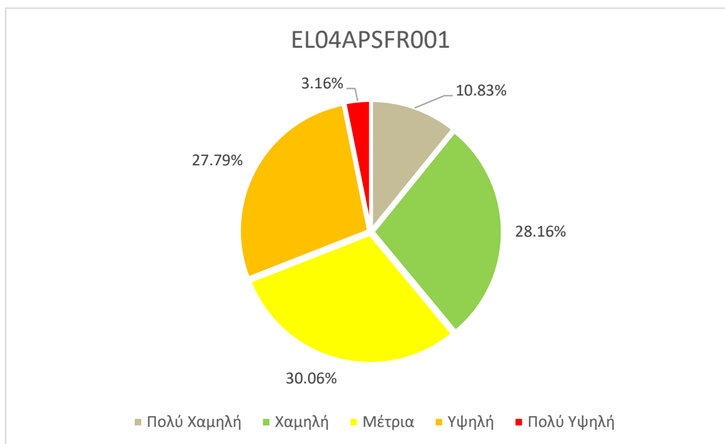
Εικόνα 3-67 Ποσοστό της συνολικής ζώνης κατάκλυσης ανά κατηγορία τρωτότητας για τη EL04APSFR001
