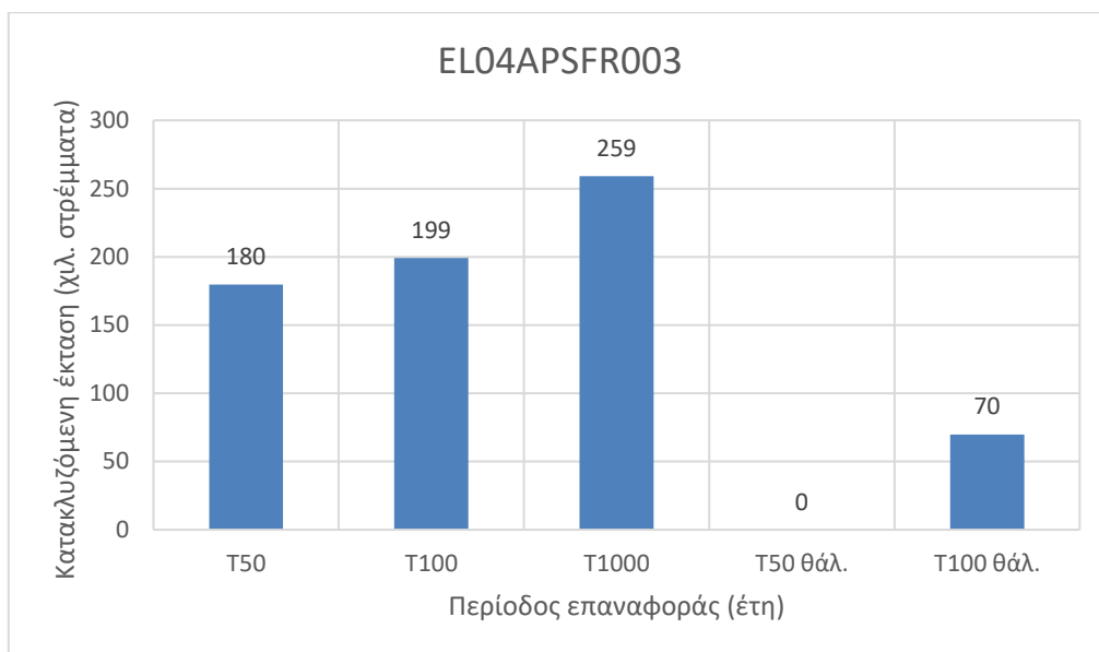
Εικόνα 3-26 Κατακλυζόμενες εκτάσεις στη EL04APSFR003 για τις πλημμύρες περιόδου επαναφοράς 50, 100 και 1 000 ετών
