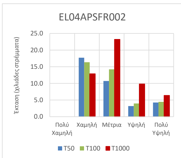
Εικόνα 3-71 Έκταση που αντιστοιχεί σε κάθε κατηγορία επικινδυνότητας πλημμύρας, ανά περίοδο επαναφοράς για τη EL04APSFR002
