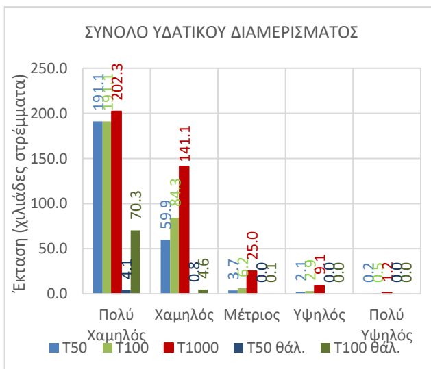
Εικόνα 3-66 Έκταση που αντιστοιχεί σε κάθε κατηγορία κινδύνου πλημμύρας, ανά περίοδο επαναφοράς για το σύνολο του ΥΔ Δυτικής Στερεάς Ελλάδας
