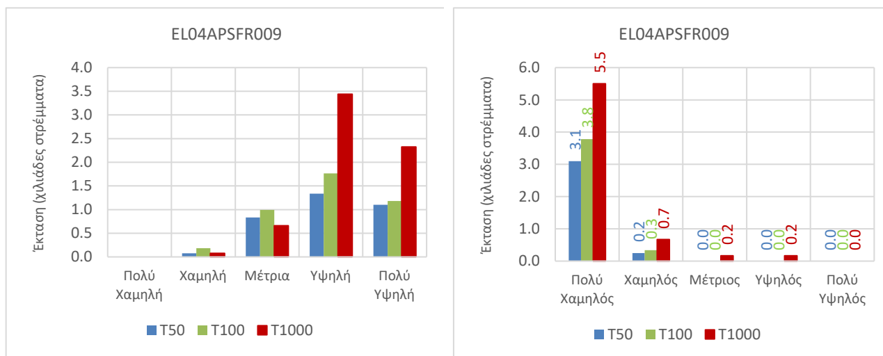
Εικόνα 3-92 Έκταση που αντιστοιχεί σε κάθε κατηγορία επικινδυνότητας πλημμύρας, ανά περίοδο επαναφοράς για τη ΖΩΝΗ EL04APSFR009
