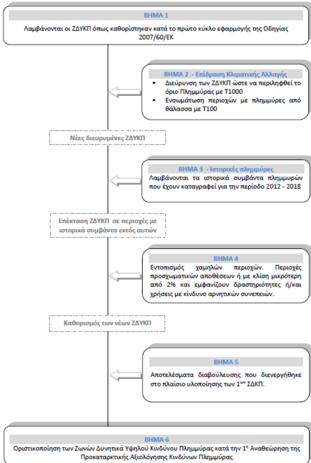
Εικόνα 3-8 Σχηματοποιημένη παρουσίαση της προσέγγισης αναθεώρησης των ΖΔΥΚΠ
