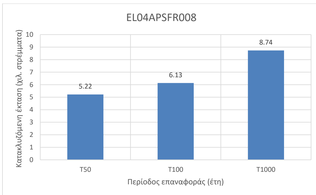
Εικόνα 3-36 Κατακλυζόμενες εκτάσεις για τις πλημμύρες περιόδου επαναφοράς 50, 100 και 1.000 ετών στη EL04APSFR008
