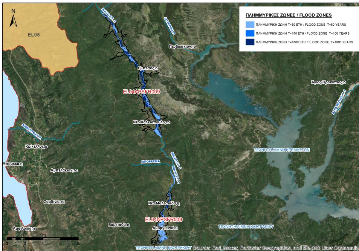
Εικόνα 3-39 Ζώνες κατάκλυσης για T=50 , T=100 και T=1000 έτη για την EL04APSFR009
