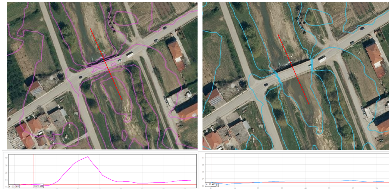
Εικόνα 3-9: Περιοχή στην οποία πραγματοποιήθηκε επεξεργασία του DTM και η αντίστοιχη τομή της. Η μορφή της περιοχής πριν την επεξεργασία απεικονίζεται με magenta.
