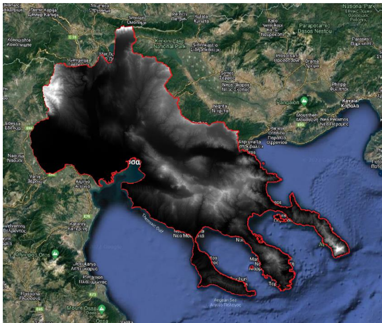
Εικόνα 3-13: Τελική μορφή ψηφιακού μοντέλου εδάφους
