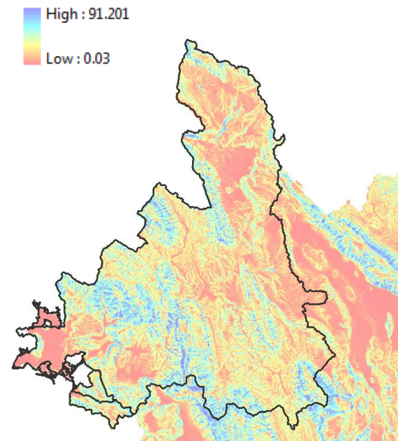
Εικόνα 4.10: Χάρτης Τοπογραφικού Συντελεστή (LS) στην λεκάνη του άνω και κάτω ρου Καλαμά
