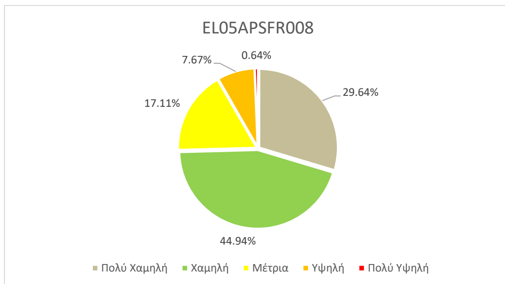
Εικόνα 3.98: Ποσοστό της συνολικής ζώνης κατάκλυσης ανά κατηγορία κινδύνου πλημμύρας (Αποτίμηση επιπτώσεων πλημμύρας), για περίοδο επαναφοράς T=100 έτη στη EL05APSFR008
