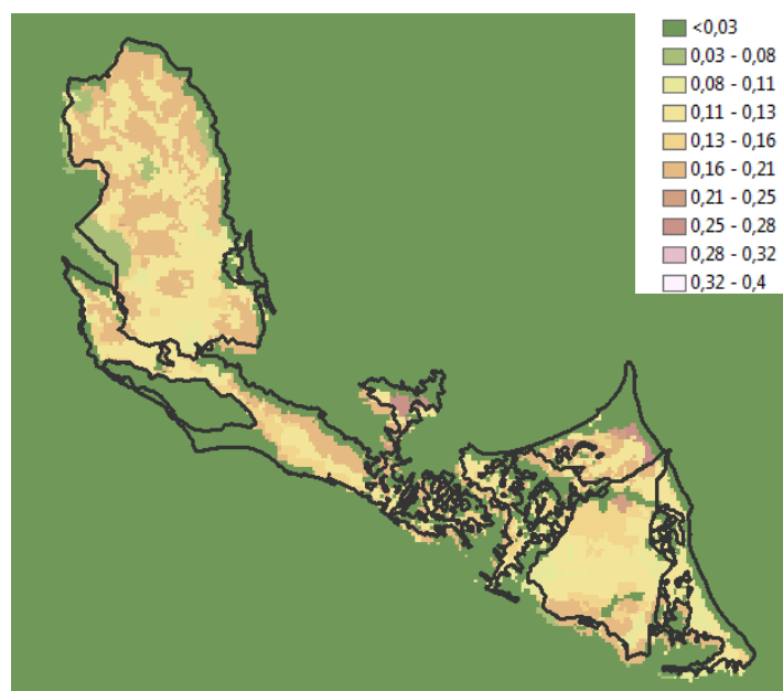
Εικόνα 4.34: Χάρτης συντελεστή φυτοκάλυψης (C) στη ΛΑΠ Κέρκυρας - Παξών
