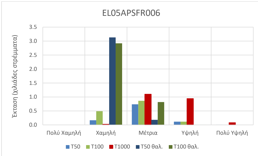
Εικόνα 3.66: Έκταση που αντιστοιχεί σε κάθε κατηγορία επικινδυνότητας πλημμύρας (Βαθμός επιρροής πλημμύρας), ανά περίοδο επαναφοράς στη EL05APSFR006
