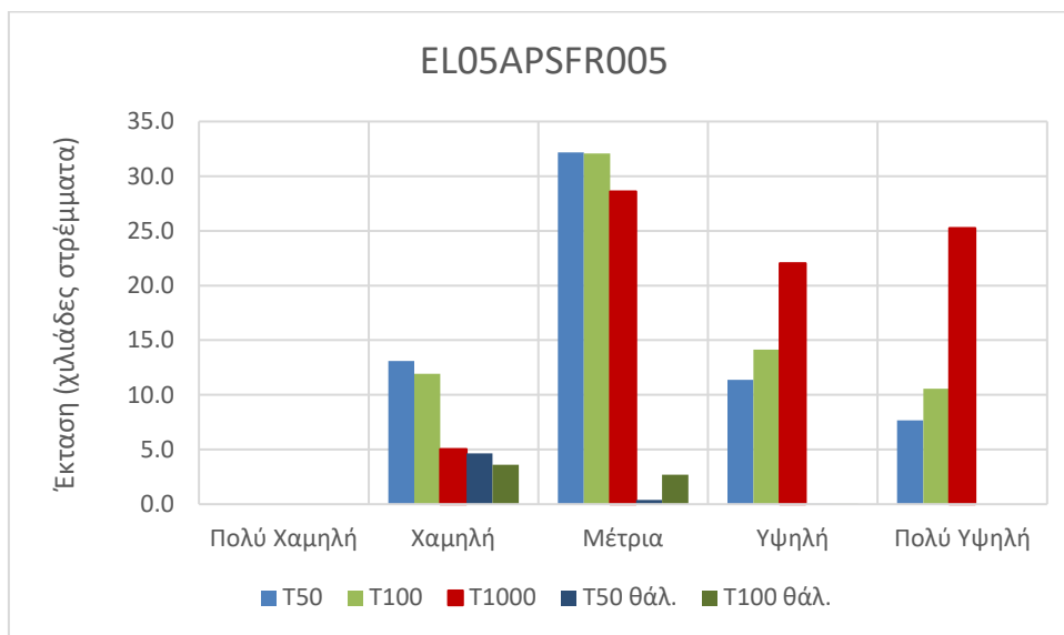
Εικόνα 3.51: Έκταση που αντιστοιχεί σε κάθε κατηγορία επικινδυνότητας πλημμύρας (Βαθμός επιρροής πλημμύρας), ανά περίοδο επαναφοράς στη EL05APSFR005
