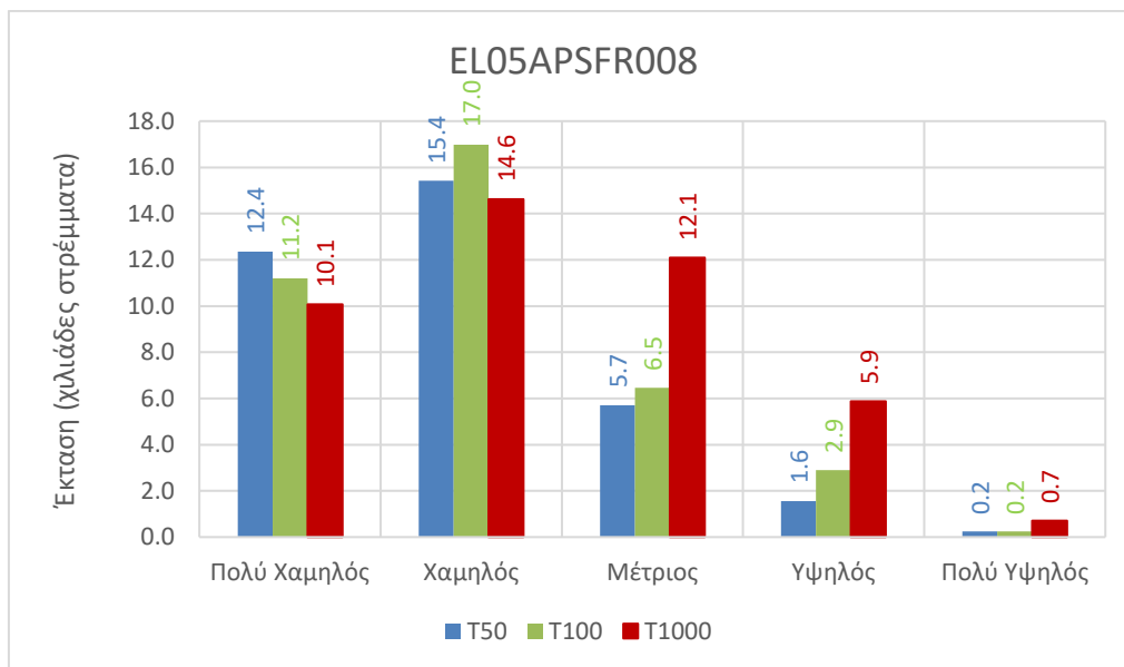
Εικόνα 3.96: Έκταση που αντιστοιχεί σε κάθε κατηγορία κινδύνου πλημμύρας (Αποτίμηση επιπτώσεων πλημμύρας) ανά περίοδο επαναφοράς στη EL05APSF008
