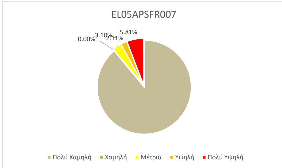
Εικόνα 3.83: Ποσοστό της συνολικής ζώνης κατάκλυσης στη EL05APSFR007 ανά κατηγορία επικινδυνότητας πλημμύρας (βαθμός επιρροής πλημμύρας), για περίοδο επαναφοράς T=50 έτη.
