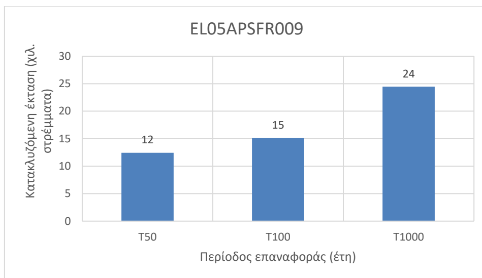
Εικόνα 3.101: Κατακλυζόμενες εκτάσεις για τις πλημμύρες περιόδου επαναφοράς 50, 100 και 1.000 ετών στη EL05APSFR009
