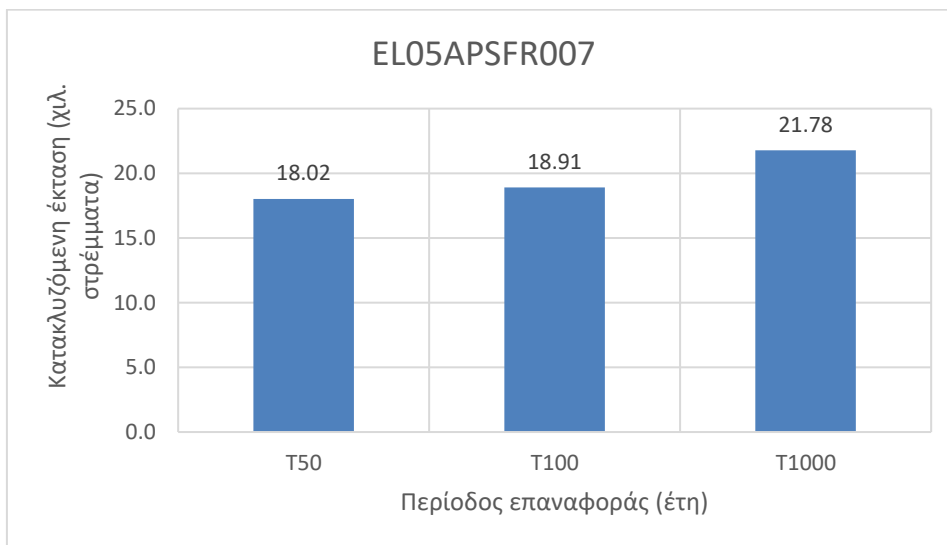
Εικόνα 3.78: Κατακλυζόμενες εκτάσεις για τις πλημμύρες περιόδου επαναφοράς 50, 100 και 1.000 ετών στη EL05APSFR007
