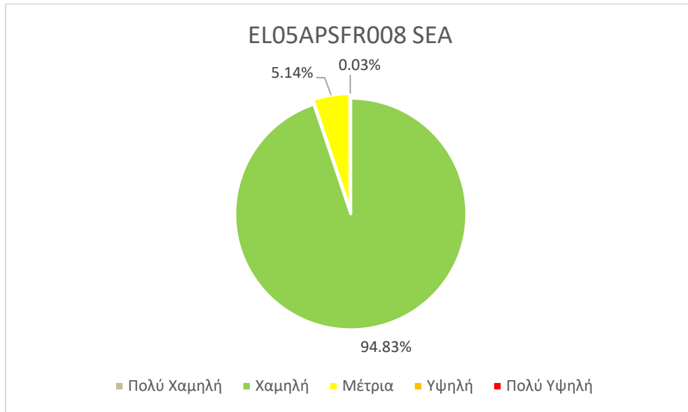
Εικόνα 3.95: Ποσοστό της συνολικής ζώνης κατάκλυσης στη EL05APSF008 ανά κατηγορία επικινδυνότητας θαλάσσιας πλημμύρας (βαθμός επιρροής πλημμύρας), για περίοδο επαναφοράς T=100 έτη
