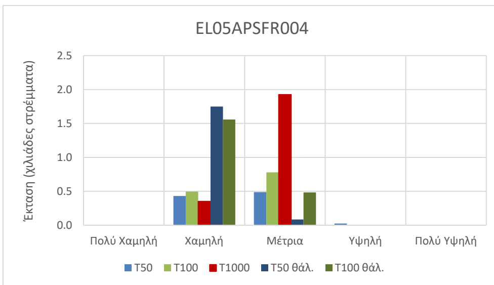
Εικόνα 3.36: Έκταση που αντιστοιχεί σε κάθε κατηγορία επικινδυνότητας πλημμύρας (Βαθμός επιρροής πλημμύρας), ανά περίοδο επαναφοράς στη EL05APSFR004
