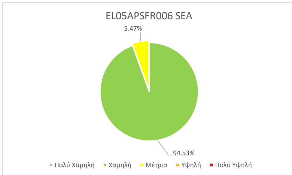
Εικόνα 3.71: Ποσοστό της συνολικής ζώνης κατάκλυσης στη EL05APSFR006 ανά κατηγορία επικινδυνότητας θαλάσσιας πλημμύρας (βαθμός επιρροής πλημμύρας), για περίοδο επαναφοράς T=50 έτη.
