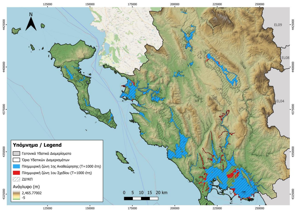
Εικόνα 6-5 Έκταση πλημμύρας 1ης Αναθεώρησης ΣΔΚΠ (μπλε χρώμα) και η έκταση πλημμύρας από 1ο κύκλο για T=1000 έτη που εκτείνεται πέρα από εκείνη της 1ης Αναθεώρησης (κόκκινο χρώμα)
