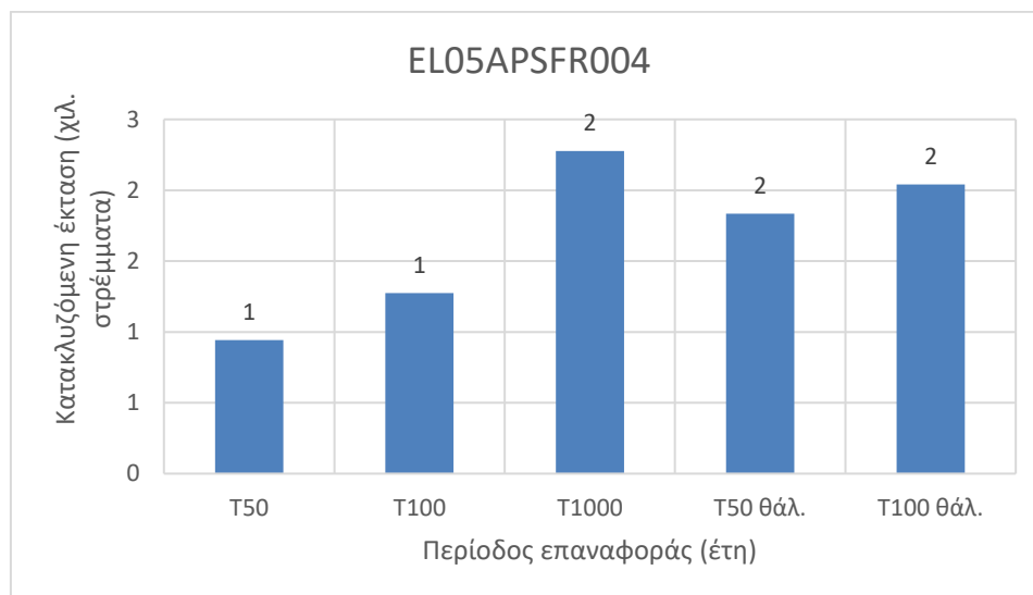
Εικόνα 3.33: Κατακλυζόμενες εκτάσεις για τις πλημμύρες περιόδου επαναφοράς 50, 100 και 1.000 ετών καθώς και για τις θαλάσσιες πλημμύρες περιόδου επαναφοράς 50 και 100 ετών στη EL05APSFR004
