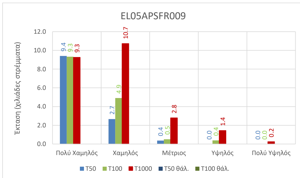
Εικόνα 3.107: Έκταση που αντιστοιχεί σε κάθε κατηγορία κινδύνου πλημμύρας (Αποτίμηση επιπτώσεων πλημμύρας) ανά περίοδο επαναφοράς στη EL05APSFR009
