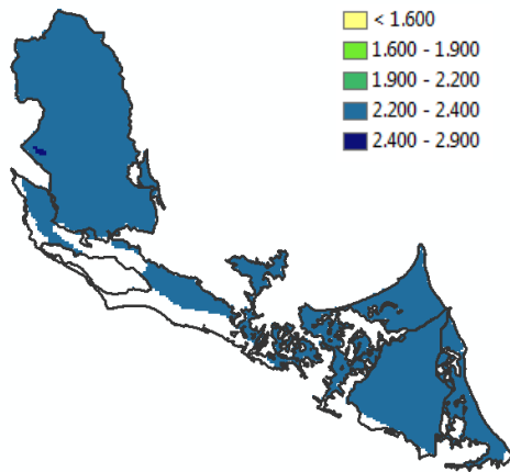
Εικόνα 4.30: Χάρτης διαβρωτικότητας της βροχόπτωσης ( R - MJ \text{ mm ha}^{-1} \text{ h}^{-1} ) στην ΛΑΠ Κέρκυρας - Παξών
