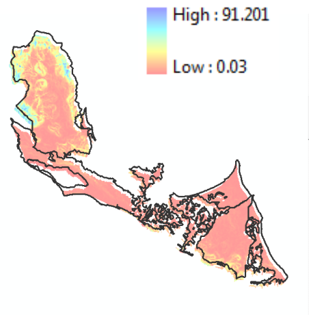
Εικόνα 4.31: Χάρτης Τοπογραφικού Συντελεστή (LS) στην ΛΑΠ Κέρκυρας - Παξών
