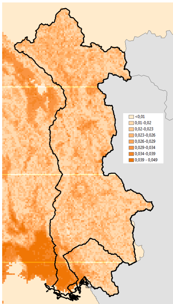
Εικόνα 4.25: Χάρτης εδαφικής διαβρωσιμότητας (K) στη ΛΑΠ Αράχθου
