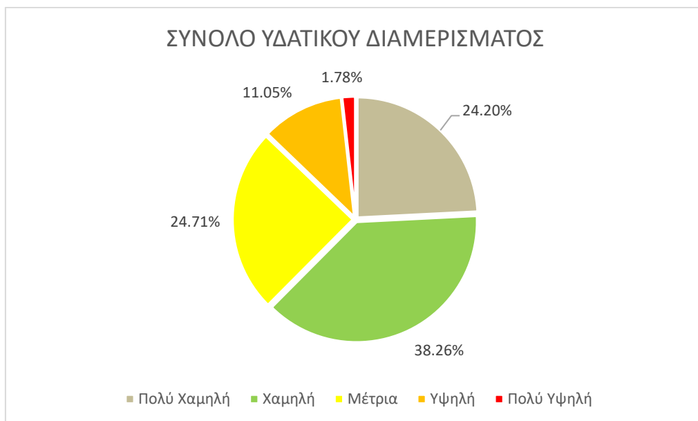
Εικόνα 3.2: Ποσοστό της συνολικής ζώνης κατάκλυσης του Υ.Δ. ανά κατηγορία τρωτότητας (Μέγιστη πιθανή επίπτωση πλημμύρας). Η συνολική ζώνη κατάκλυσης αντιστοιχεί στην πλημμύρα περιόδου επαναφοράς 1.000 ετών.
