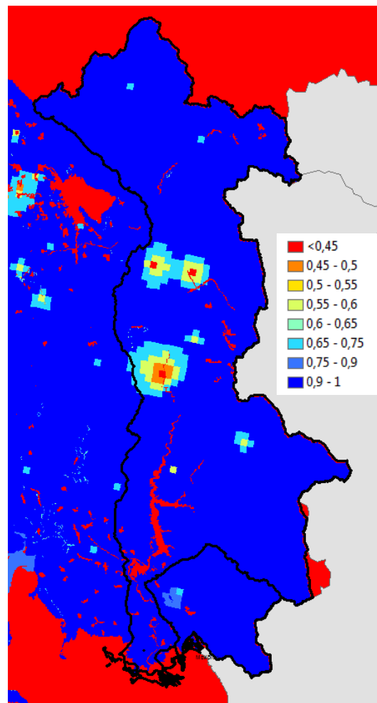
Εικόνα 4.26: Χάρτης διαχείρισης των εδαφών κατά της διάβρωσης (P) στην ΛΑΠ Αράχθου
