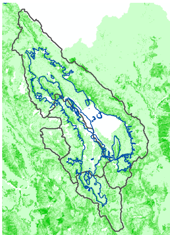
Εικόνα 4.7: Χάρτης εδαφικής απώλεια (SE) στη κλειστή λεκάνη Ιωαννίνων και της ΖΔΥΚΠ EL05APSF009 της περιοχής «Χαμηλή Ζώνη Κλειστής Λεκάνης Ιωαννίνων»
