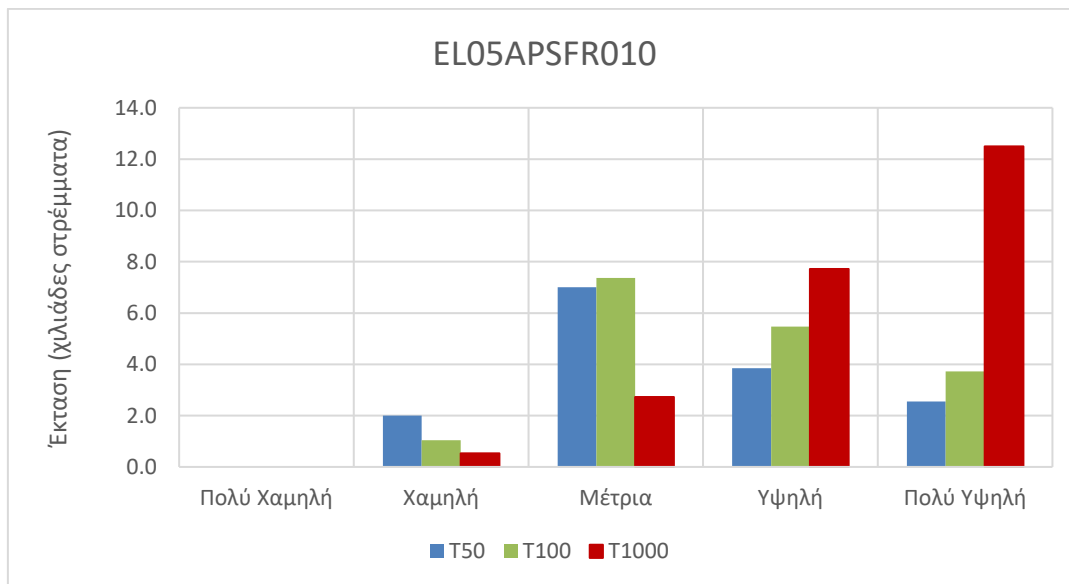
Εικόνα 3.113: Έκταση που αντιστοιχεί σε κάθε κατηγορία επικινδυνότητας πλημμύρας (Βαθμός επιρροής πλημμύρας), ανά περίοδο επαναφοράς στη EL05APSFR010
