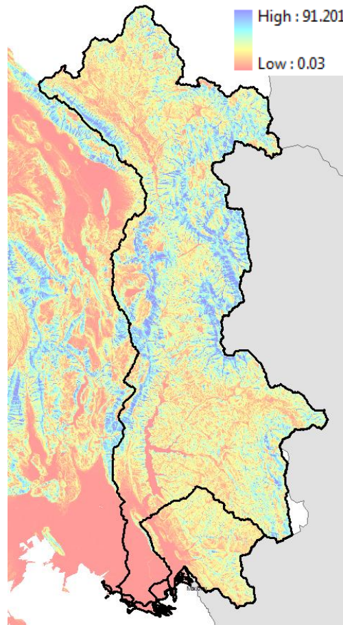
Εικόνα 4.24: Χάρτης Τοπογραφικού Συντελεστή (LS) στην ΛΑΠ Αράχθου
