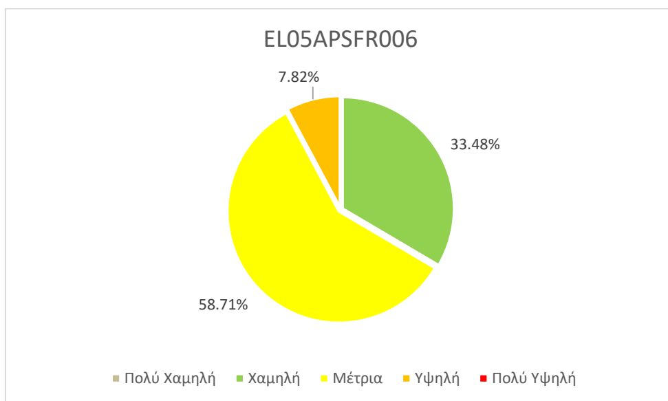
Εικόνα 3.68: Ποσοστό της συνολικής ζώνης κατάκλυσης στη EL05APSFR006 ανά κατηγορία επικινδυνότητας πλημμύρας (βαθμός επιρροής πλημμύρας), για περίοδο επαναφοράς T=100 έτη.
