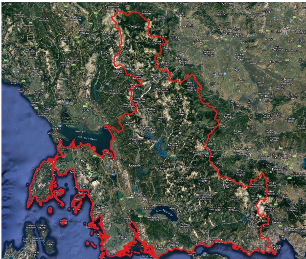
Εικόνα 3-1 Υδατικό διαμέρισμα EL04
