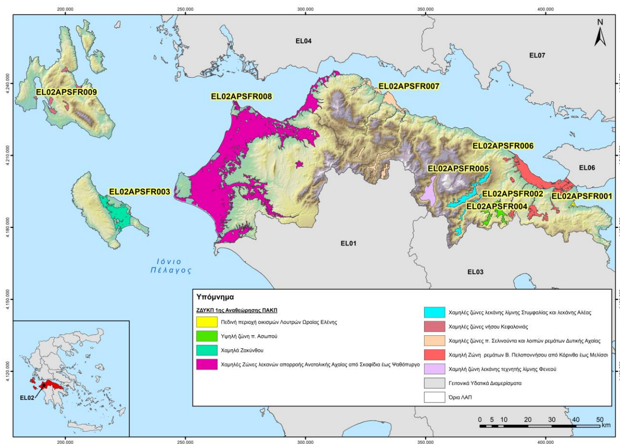
Σχήμα 2.6: Ζώνες Δυνητικά Υψηλού Κινδύνου Πλημμύρας της 1ης Αναθεώρησης της ΠΑΚΠ για το ΥΔ Βόρειας Πελοποννήσου
