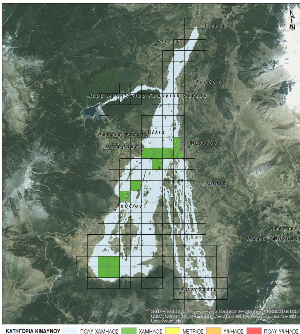
Σχήμα 3.7 : Αξιολόγηση επιπτώσεων πλημμύρας για T=100 έτη - ΖΔΥΚΠ GR02RAK0005 - Χαμηλή ζώνη λεκάνης τεχνητής λίμνης Φενεού
