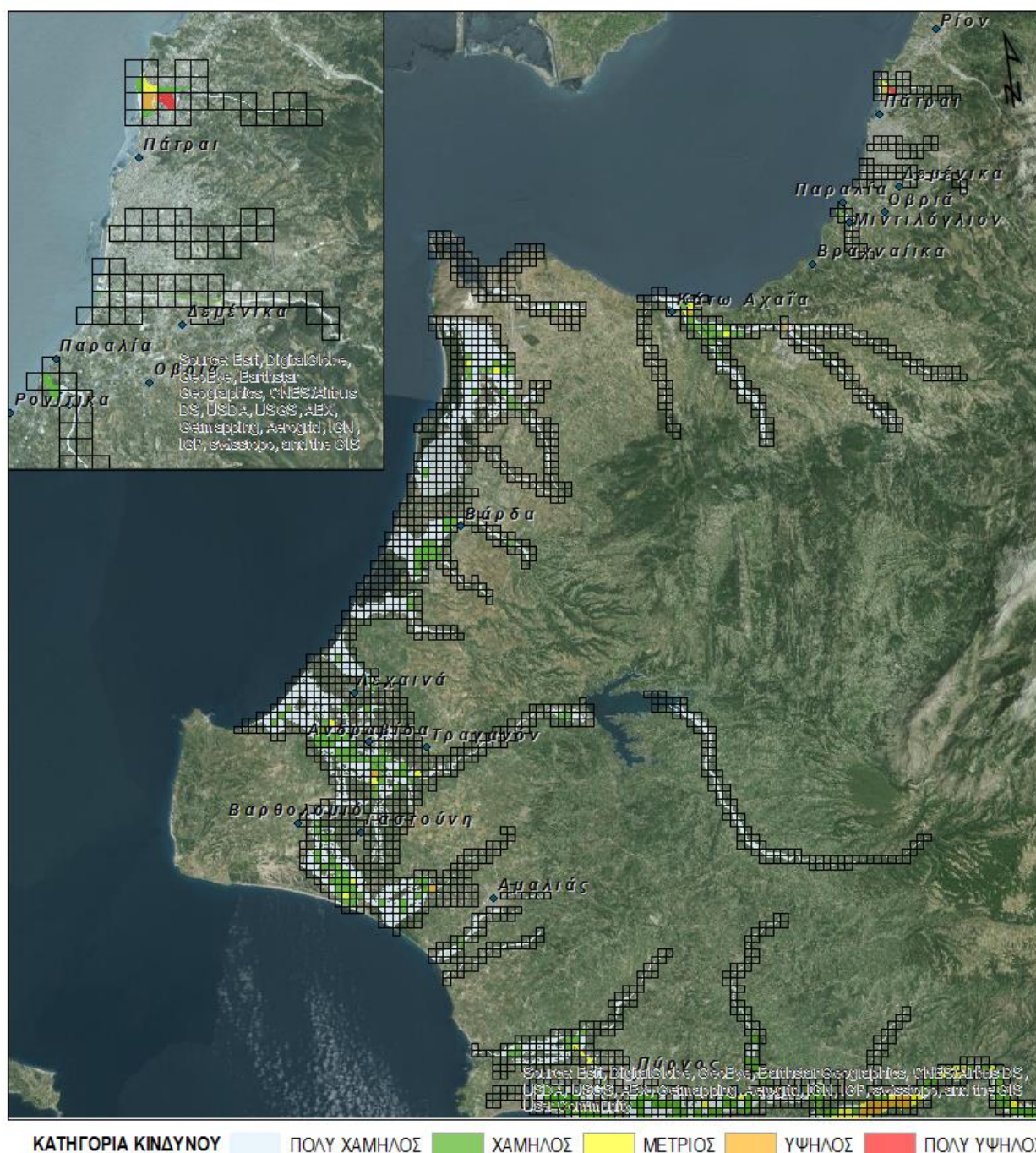
Σχήμα 3.10 : Αξιολόγηση επιπτώσεων πλημμύρας για T=100 έτη - ΖΔΥΚΠ GR02RAK0008 - Πεδινή ζώνη λεκανών απορροής Πείρου - Βέργα - Πηνειού -Γλαύκου
