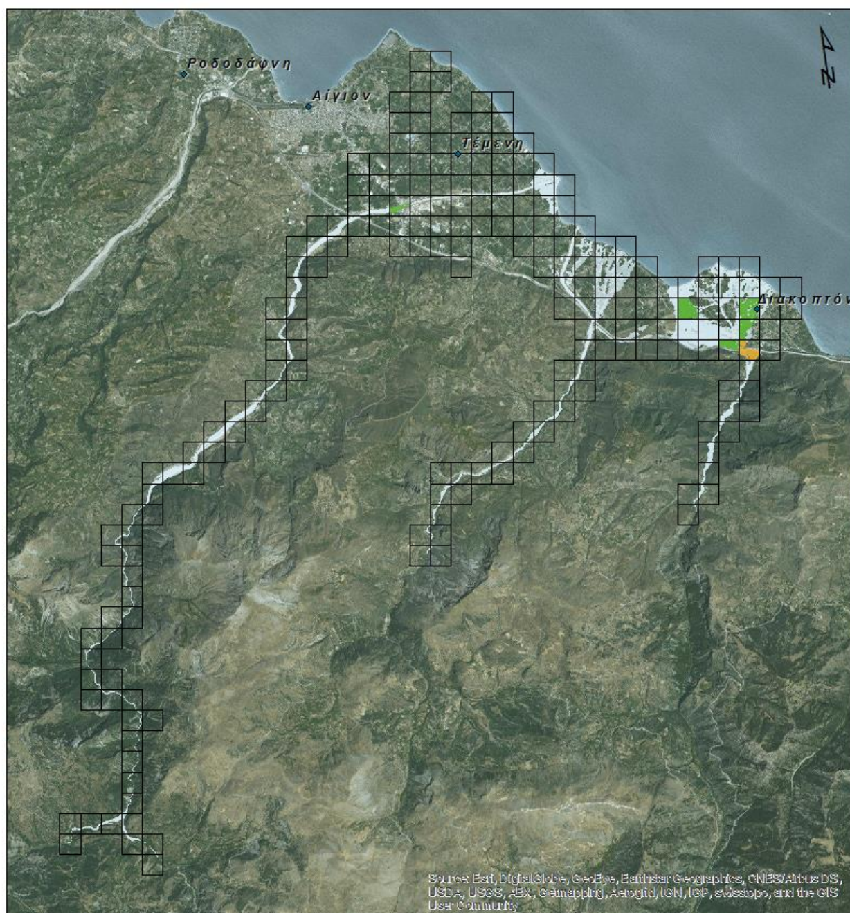
Σχήμα 3.9 : Αξιολόγηση επιπτώσεων πλημμύρας για T=100 έτη - ΖΔΥΚΠ GR02RAK0007 - Χαμηλή ζώνη π. Σελινούντα
