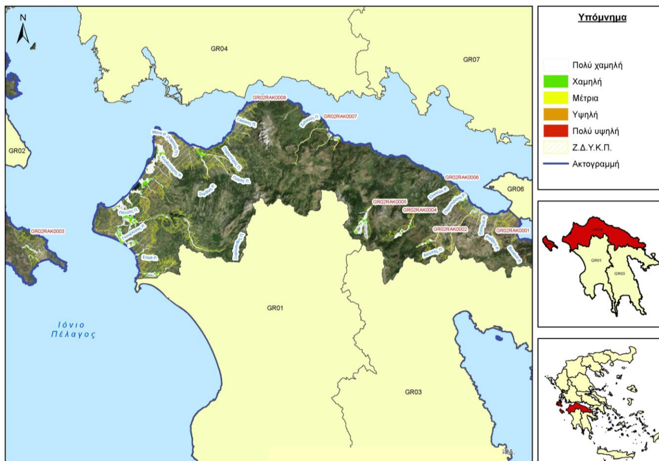
Σχήμα 3.2 : Χάρτης αποτίμησης επιπτώσεων πλημμύρας ΥΔ Βόρειας Πελοποννήσου ( T=100 έτη) για ποτάμια ροές/λίμνες
