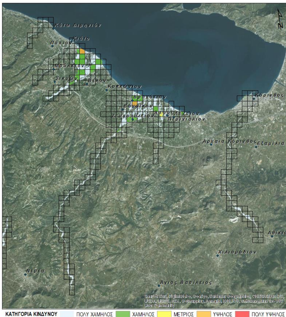
Σχήμα 3.8 : Αξιολόγηση επιπτώσεων πλημμύρας για T=100 έτη - ΖΔΥΚΠ GR02RAK0006-Χαμηλή ζώνη ρεμάτων παραλίας Β. Πελοποννήσου από το Κιάτο έως την Κόρινθο
