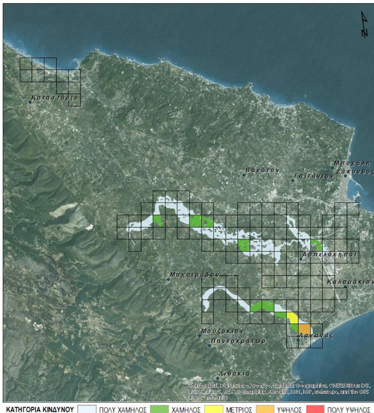
Σχήμα 3.5 : Αξιολόγηση επιπτώσεων πλημμύρας για T=100 έτη - ΖΔΥΚΠ GR02RAK0003 - Χαμηλά Ζακύνθου
