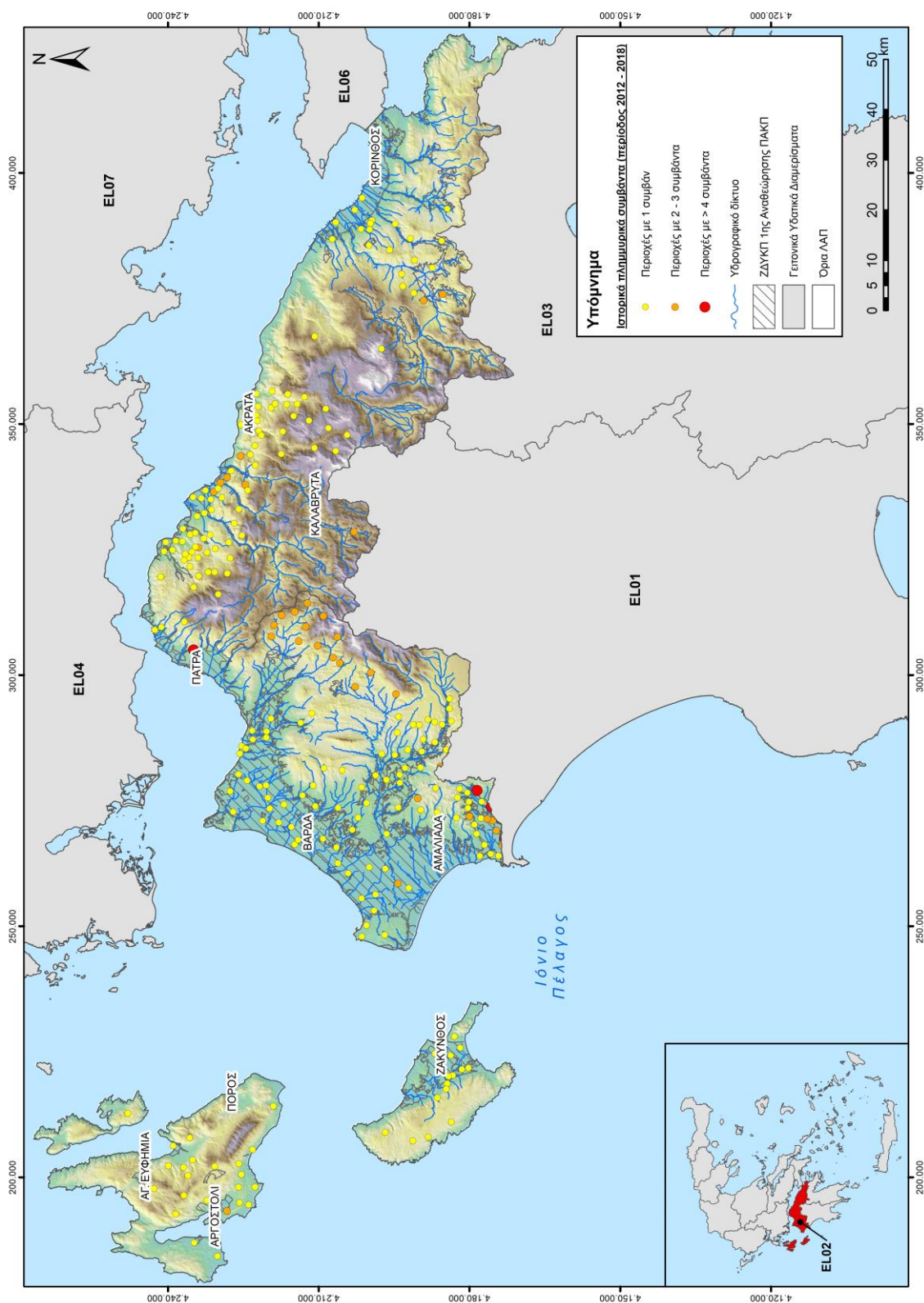
Σχήμα 2.2 : Κατηγορίες ανά αριθμό πλημμυρικών γεγονότων στις θέσεις ιστορικών πλημμυρικών συμβάντων στο ΥΔ Βόρειας Πελοποννήσου (περίοδος 2012-2018)
