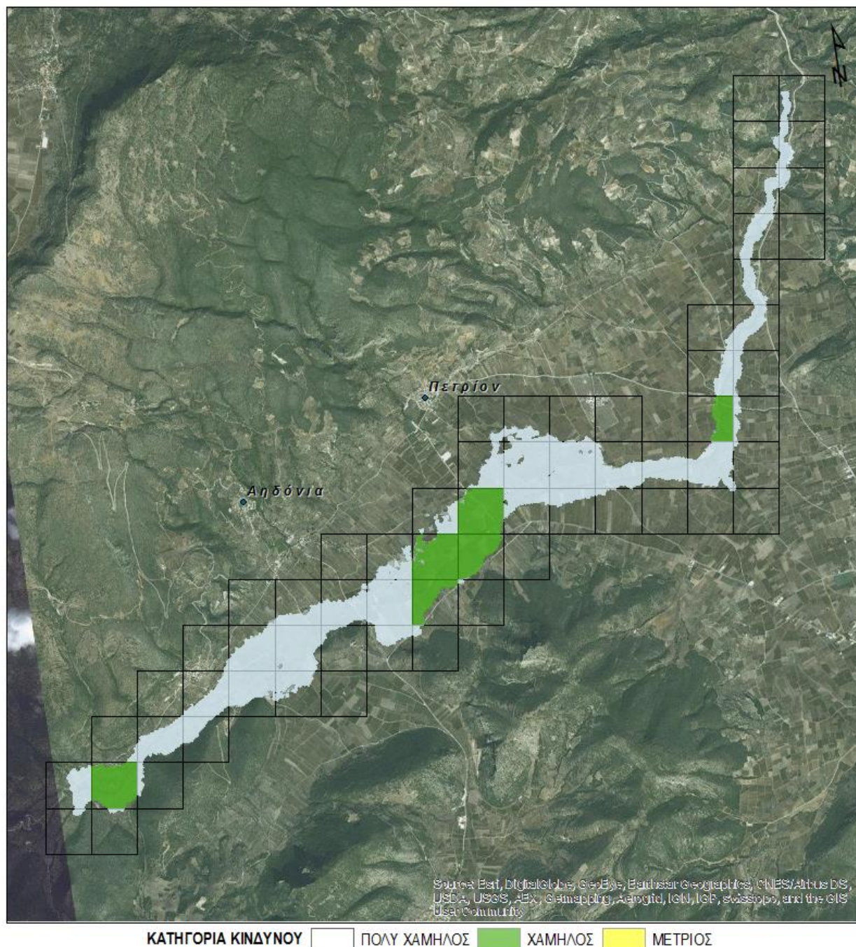
Σχήμα 3.4 : Αξιολόγηση επιπτώσεων πλημμύρας για T=100 έτη - ΖΔΥΚΠ GR02RAK0002- Υψηλή ζώνη π. Ασωπού
