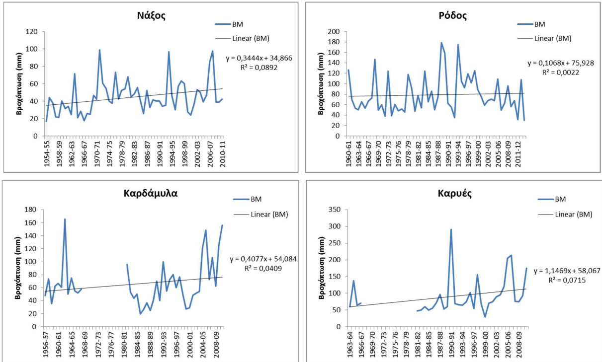
Σχήμα 4.1: Βροχομετρικοί σταθμοί στους οποίους οι χρονοσειρές των μέγιστων ημερήσιων βροχοπτώσεων εμφανίζουν ανοδικές (ή ελαφρώς ανοδικές) τάσεις.
