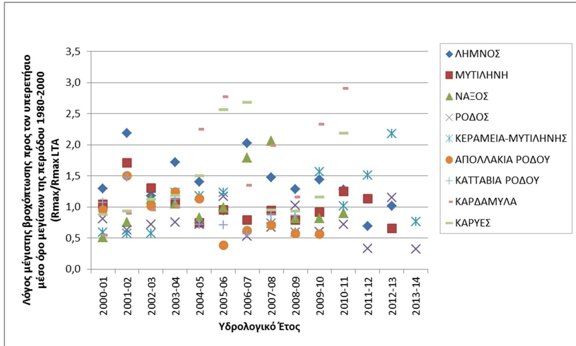
Σχήμα 4.3: Σχέση των μέγιστων ημερήσιων βροχοπτώσεων με τον υπερετήσιο μέσο όρο των μέγιστων ημερήσιων βροχοπτώσεων της περιόδου 1980-2000 ανά έτος και σταθμό ( R_{\max}^{\text{Έτους}}/R_{\max}^{\text{LTA}} )
