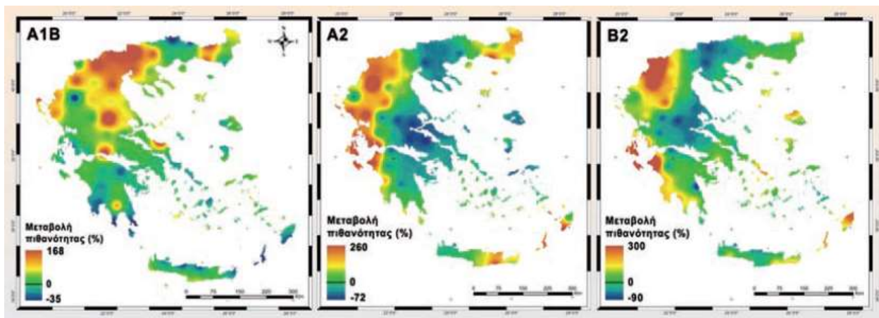
Σχήμα 4.5: Εκατοστιαία μεταβολή πιθανότητας υπέρβασης του ορίου έντασης βροχοπτώσης (threshold) πέρα από το οποίο προκύπτει αυξημένος κίνδυνος πλημμύρας μεταξύ της περιόδου ελέγχου (1960-1990) και της περιόδου 2070-2100 για τα Σενάρια A2, B2 και της περιόδου 2090-2099 για το Σενάριο A1B.
