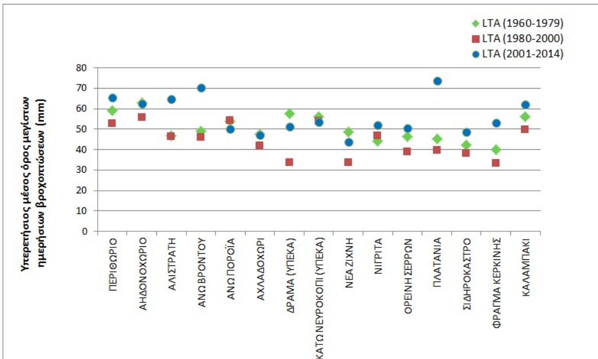
Σχήμα 4.4: Υπερετήσιο μέσοι όροι των μεγίστων ημερήσιων βροχοπτώσεων για τις περιόδους 1960-1979, 1980-2000, 2001-2014 ανά σταθμό.
