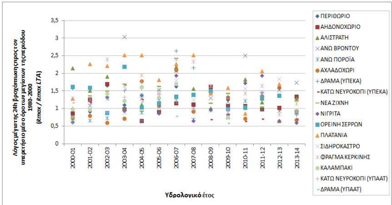
Σχήμα 4.3: Σχέση των μέγιστων ημερήσιων βροχοπτώσεων με τον υπερετήσιο μέσο όρο των μεγίστων ημερήσιων βροχοπτώσεων της περιόδου 1980-2000 ανά έτος και σταθμό ( R_{max} \text{ Έτους} / R_{maxLTA} )
