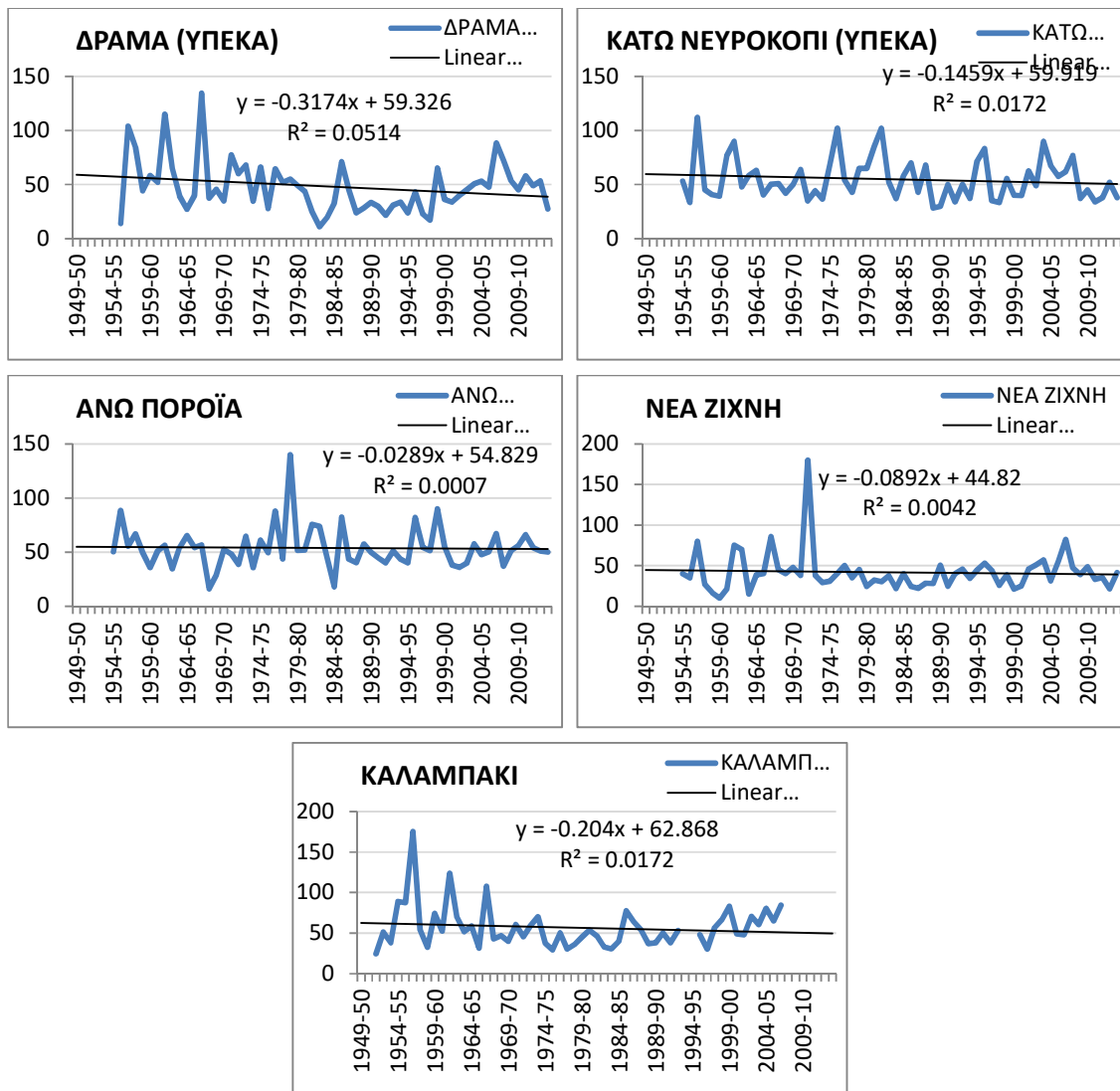
Σχήμα 4.2: Βροχομετρικοί σταθμοί στους οποίους οι χρονοσειρές των μέγιστων ημερήσιων βροχοπτώσεων εμφανίζουν πτωτικές (ή ελαφρώς πτωτικές) τάσεις.
