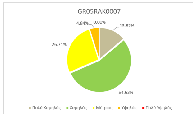
Εικόνα 10.2: Ποσοστό της συνολικής ζώνης κατάκλυσης ανά κατηγορία τρωτότητας. Η συνολική ζώνη κατάκλυσης αντιστοιχεί στην πλημμύρα περιόδου επαναφοράς 1.000 ετών
