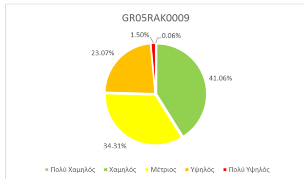
Εικόνα 12.2: Ποσοστό της συνολικής ζώνης κατάκλυσης ανά κατηγορία τρωτότητας. Η συνολική ζώνη κατάκλυσης αντιστοιχεί στην πλημμύρα περιόδου επαναφοράς 1.000 ετών.
