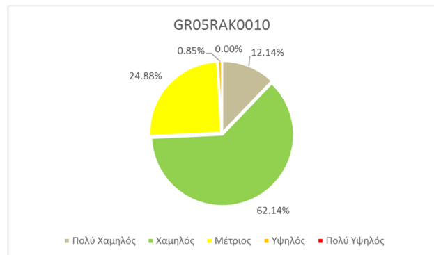
Εικόνα 13.2: Ποσοστό της συνολικής ζώνης κατάκλυσης ανά κατηγορία τρωτότητας. Η συνολική ζώνη κατάκλυσης αντιστοιχεί στην πλημμύρα περιόδου επαναφοράς 1.000 ετών.
