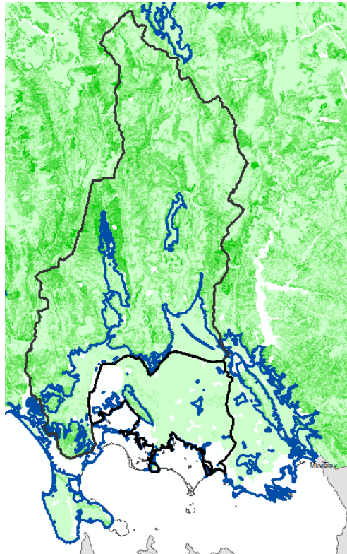
Εικόνα 14.6: Χάρτης εδαφικής απώλεια (SE) στη λεκάνη απορροής του Λούρου, της ΖΔΥΚΠ «Πεδιάδες Άρτας, Χαμηλή Ζώνη π. Λούρου & Αράχθου - GR05RAK0003» και της ΖΔΥΚΠ «Μέσος Ρους π. Λούρου - GR05RAK0001»
