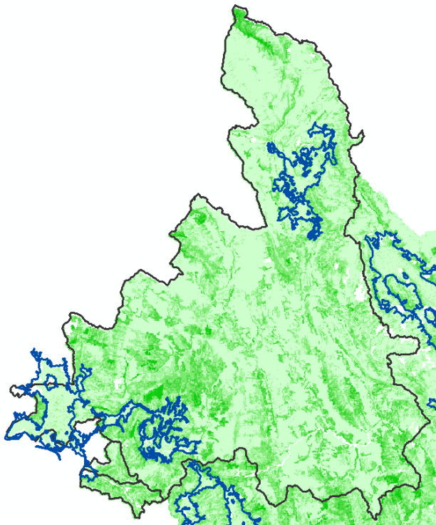
Εικόνα 14.2: Χάρτης εδαφικής απώλειας (SE) στην υδρολογική λεκάνη του άνω και κάτω ρου Καλαμά και των ΖΔΥΚΠ «Χαμηλή Περιοχή Άνω Ρου ποταμού Καλαμά στην περιοχή Δολιανά – GR05RAK0010», «Μέσος Ρους Καλαμά από το Ύψος της Βροσίνας έως το Καστρί – GR05RAK0007» και «Κάτω Ρου – Δέλτα Π. Καλαμά και Παράκτια Ζώνη Ηγουμενίτσας – GR05RAK0008»
