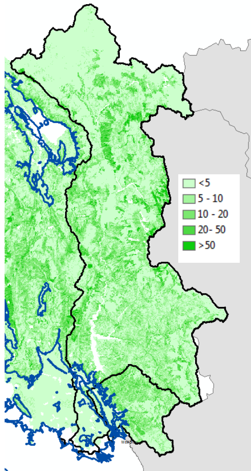
Εικόνα 14.4: Χάρτης εδαφικής απώλειας (SE) στη λεκάνη απορροής του Αράχθου και της ΖΔΥΚΠ GR05RAK0003
