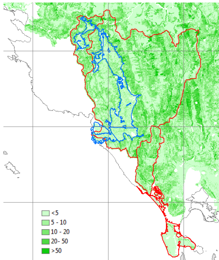
Εικόνα 14.3: Χάρτης εδαφικής απώλειας (SE) στη λεκάνη απορροής του Αχέροντα, της ΖΔΥΚΠ GR05RAK0005 της περιοχής. Χαμηλές Περιοχές Λεκάνης ποταμού Αχέροντα και κλειστής λεκάνης Μαργαριτίου και της ΖΔΥΚΠ GR05RAK0002.
