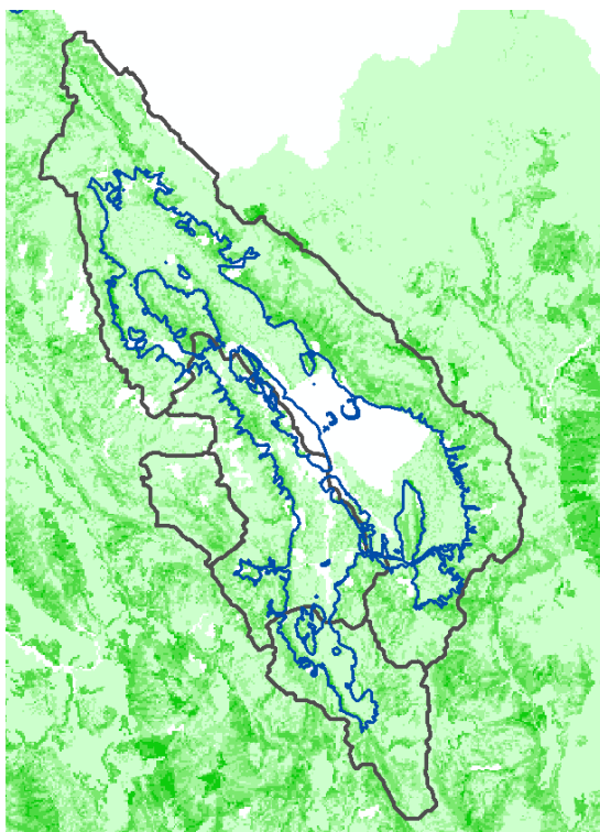
Εικόνα 14.1: Χάρτης εδαφικής απώλειας (SE) στη κλειστή λεκάνη Ιωαννίνων και της ΖΔΥΚΠ GR05RAK0009 της περιοχής «Χαμηλή Ζώνη Κλειστής Λεκάνης Ιωαννίνων»
