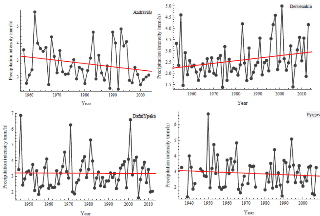
Εικόνα 4.1: Παραδείγματα προσαρμογής γραμμής τάσης σε μεγάλοι μήκους δείγματα μέγιστων ημερήσιων υψών βροχής (πάνω αριστερά: Ανδραβίδα, πτωτική τάση, πάνω δεξιά:
