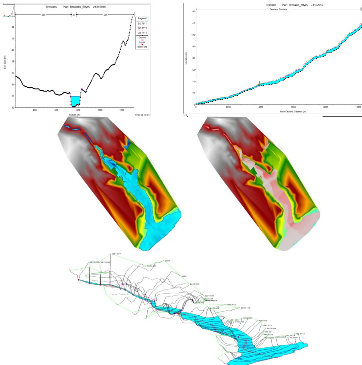
Σχήμα 5.8: Σχηματική απεικόνιση αποτελεσμάτων που εξάγονται από μοντέλο διάδρασης πλημμύρας
