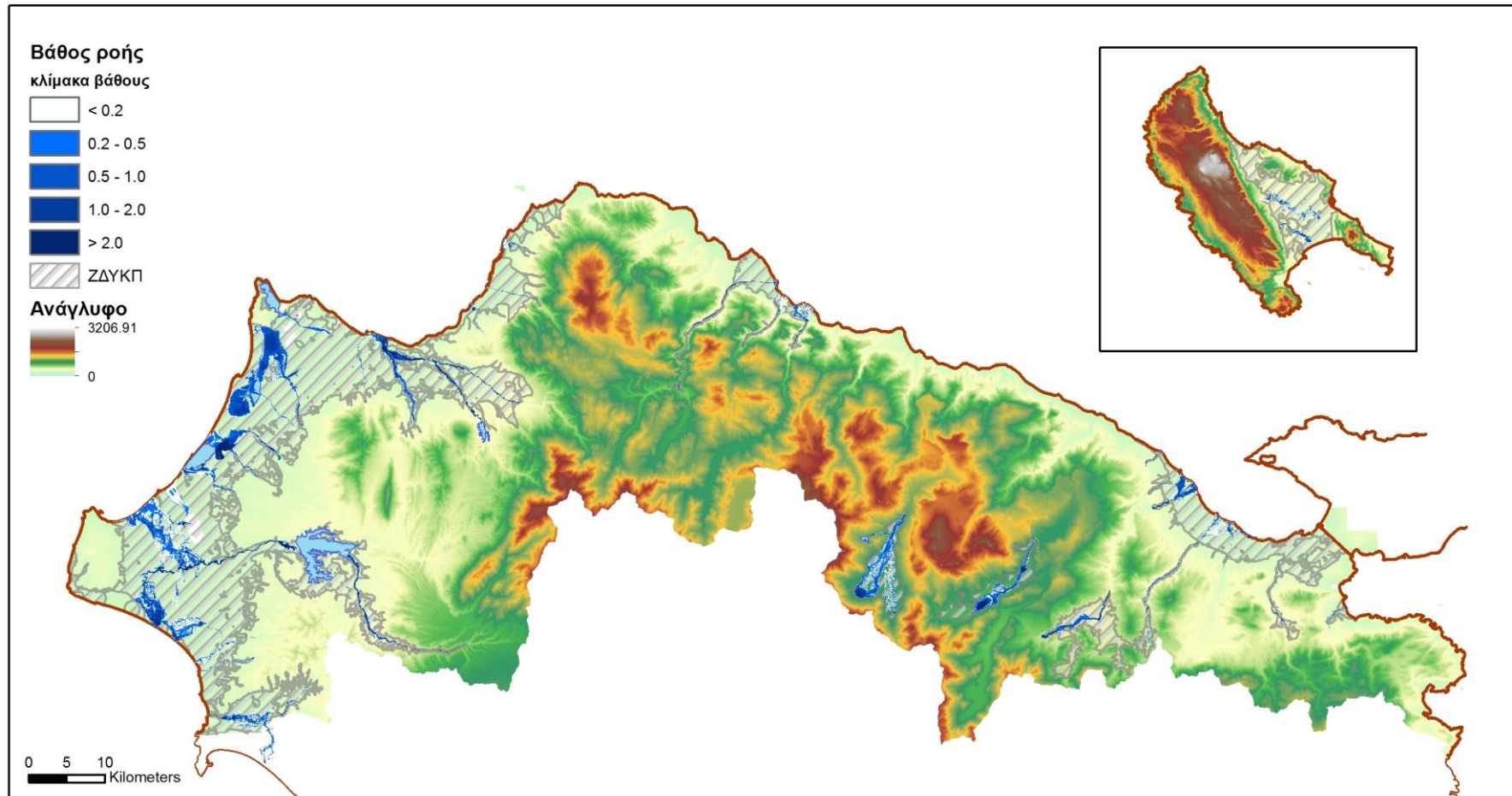
Σχήμα 6.4: Σχηματική απεικόνιση αποτελεσμάτων βάθους ροής του μοντέλου διάδευσης πλημμύρας για T=100 έτη στο Υδατικό Διαμέρισμα Βόρειας Πελοποννήσου (ΥΔ 02)
