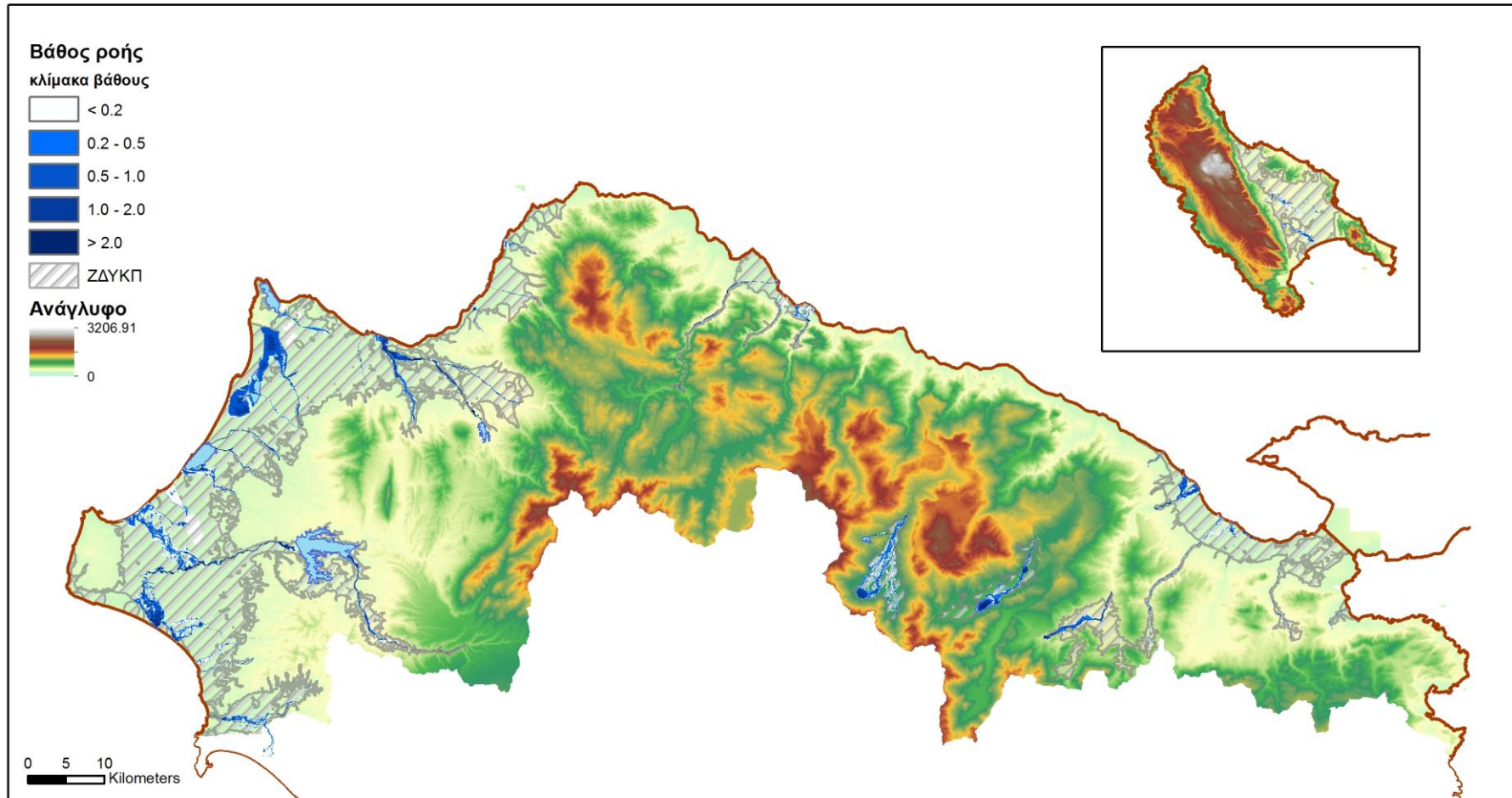
Σχήμα 6.3: Σχηματική απεικόνιση αποτελεσμάτων βάθους ροής του μοντέλου διάδρασης πλημμύρας για T=50 έτη στο Υδατικό Διαμέρισμα Βόρειας Πελοποννήσου (ΥΔ 02)
