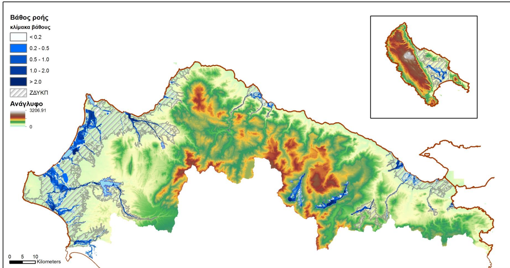
Σχήμα 6.5: Σχηματική απεικόνιση αποτελεσμάτων βάθους ροής του μοντέλου διάδευσης πλημμύρας για T=1000 έτη στο Υδατικό Διαμέρισμα Βόρειας Πελοποννήσου (ΥΔ 02)
