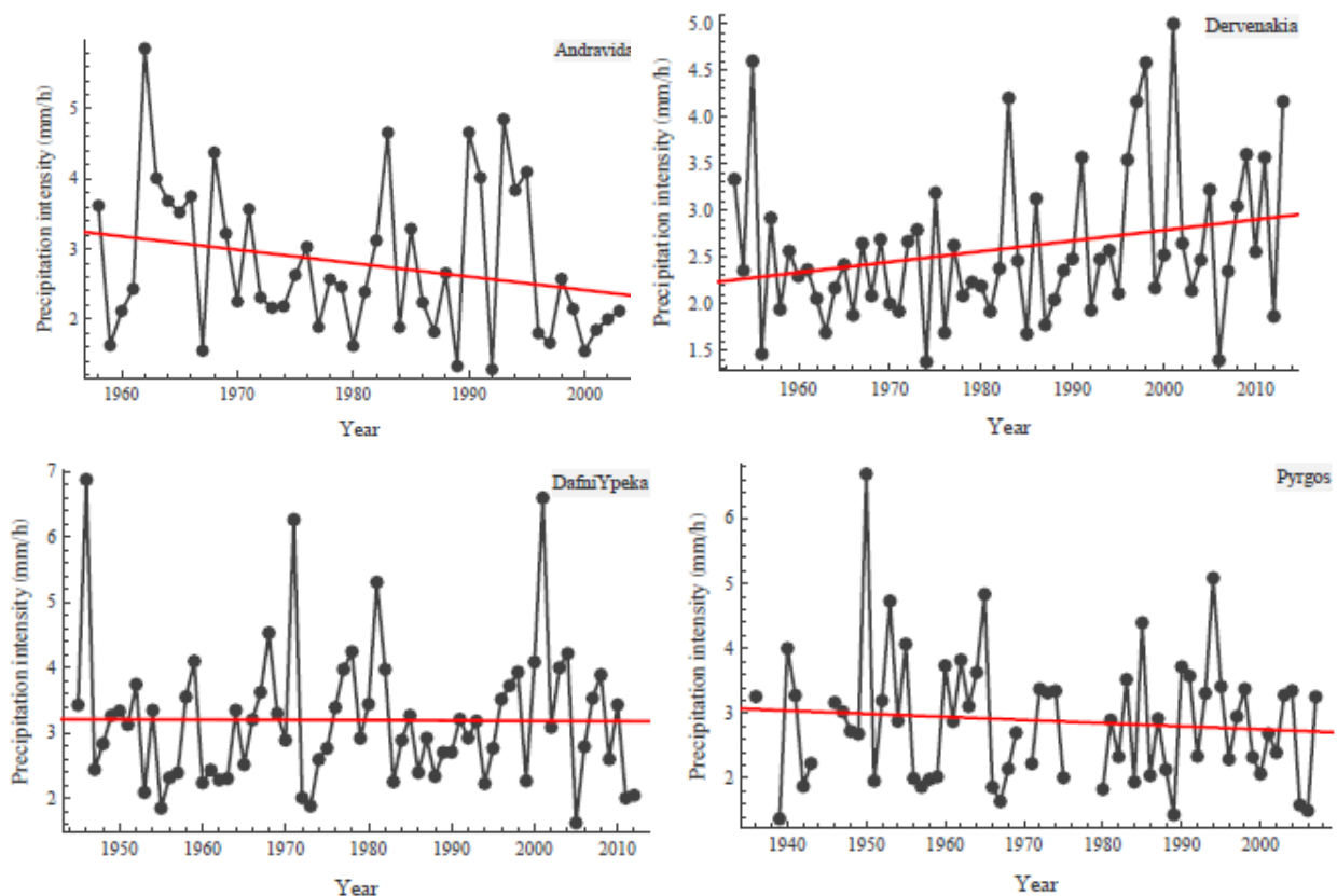
Εικόνα 4.1: Παραδείγματα προσαρμογής γραμμής τάσης σε μεγάλο μήκος δείγματα μέγιστων ημερήσιων υψών βροχής (πάνω αριστερά: Ανδραβίδα, πτωτική τάση, πάνω δεξιά:
